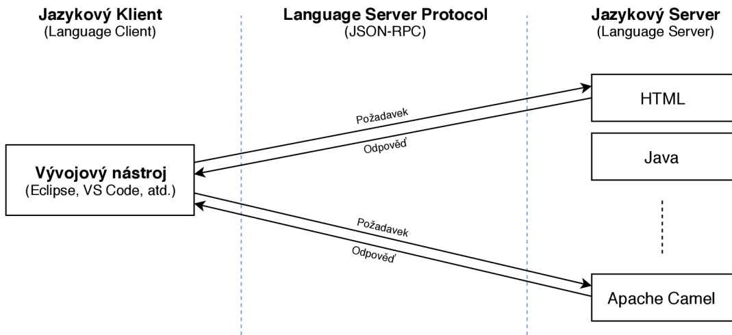
Obr. 1.2: Ukázka podpory více jazykových serverů současně.
