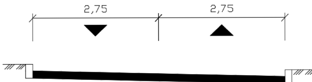
Obr. 3 Příčné uspořádání dvoupruhové komunikace MO2 5,8/5,5/30
