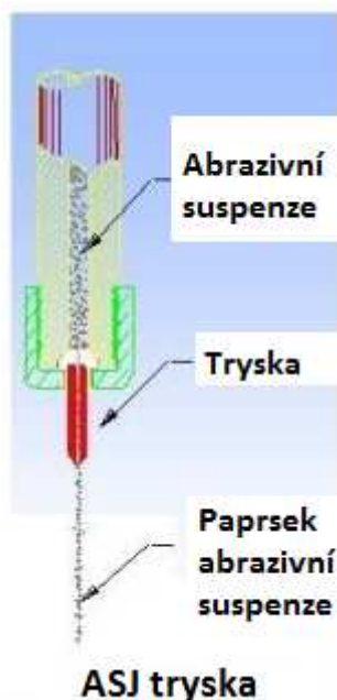
Obr. 1.33 ASJ tryska [6]
