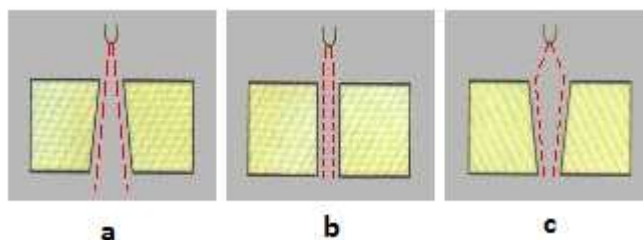
Obr. 3.12 Tvary úkosů [17]
