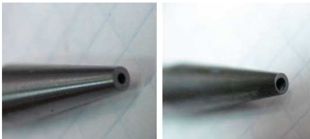
Obr. 2.22 Opotřebení zaměřovací abrazivní trysky[12]
