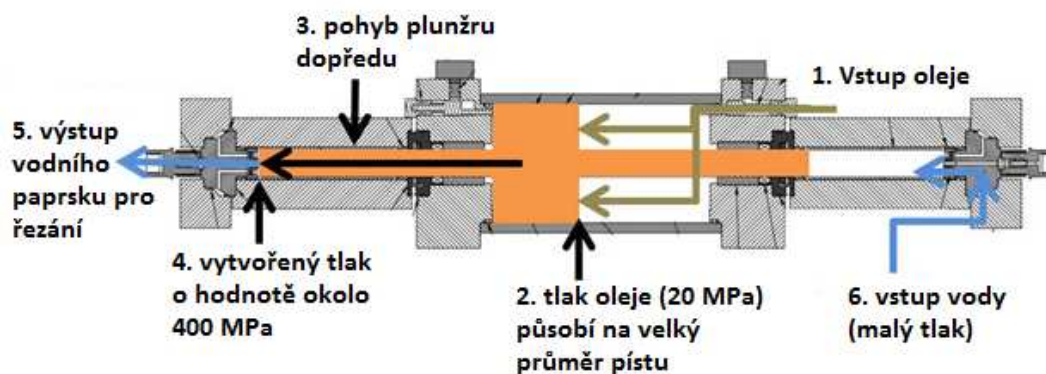
Obr. 2.13 Princip multiplikátoru[11]
