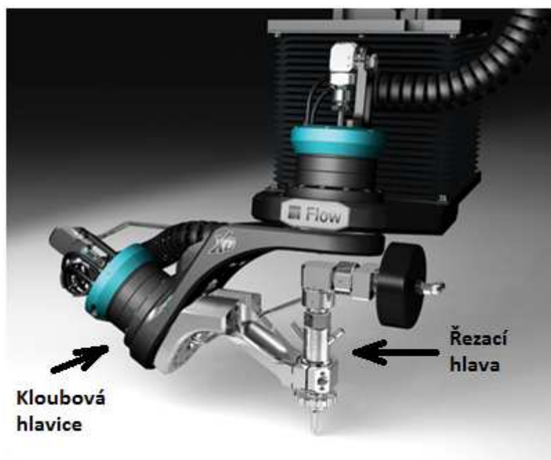
Obr. 1.35 DWJ Řezná hlavice XD
