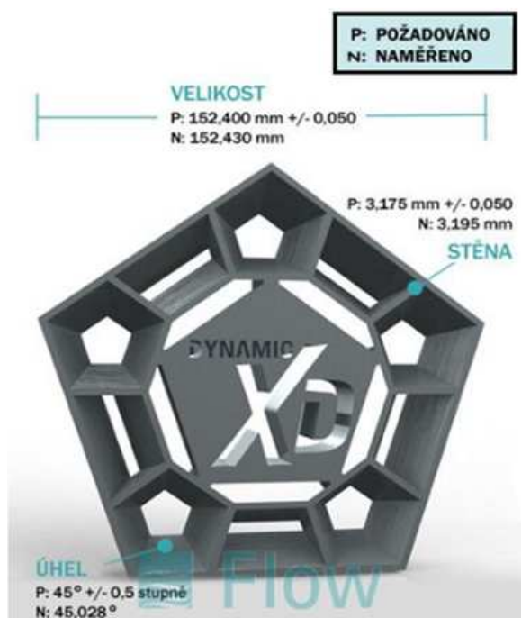
Obr. 4.22 Zhotovený dílec technologií DWJXD [5]
