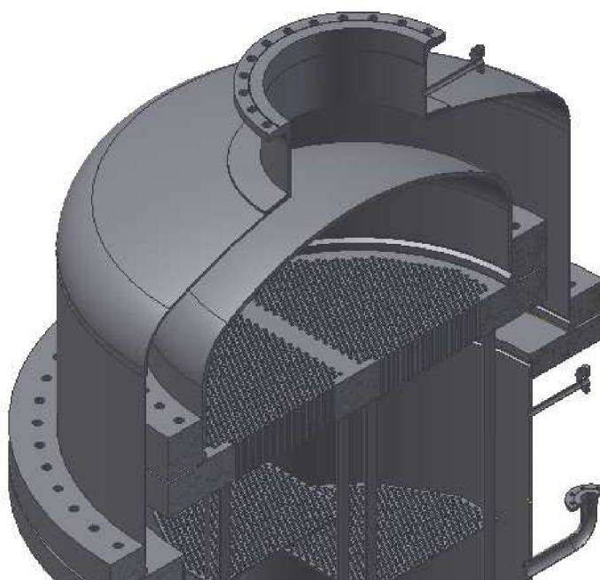
Obr. 4-13 Výměník s plovoucí hlavou (pracovní pozice)
