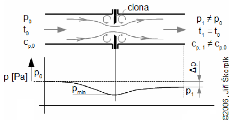
Obr. 3-2 Škrčení páry, [2]
