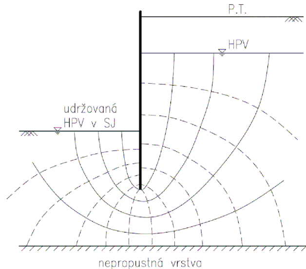
Obr. 6-2: Proudová síť- proudnice – plné čáry, ekvipotenciály – čárkovaná čára
