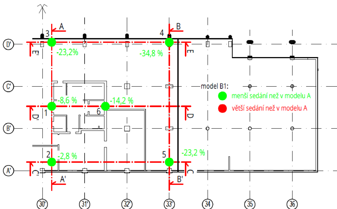
Obr. 6-14: Finální srovnání sedání v podobě procentuálních rozdílů v poslední fázi č. 12, model B1 vs. model A
