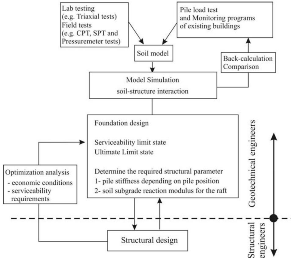
Obr. 2-7: Vývojový diagram návrhu PRF (El- Mossallamy, 2006)
