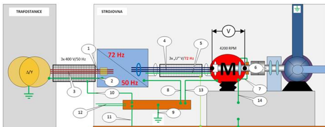
Obr. 5) Příklad diagnostiky zařízení s frekvenčním měničem
