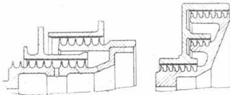
Obr. č.3.4 – Patrové uspořádání labyrintových ucpávek[5]
