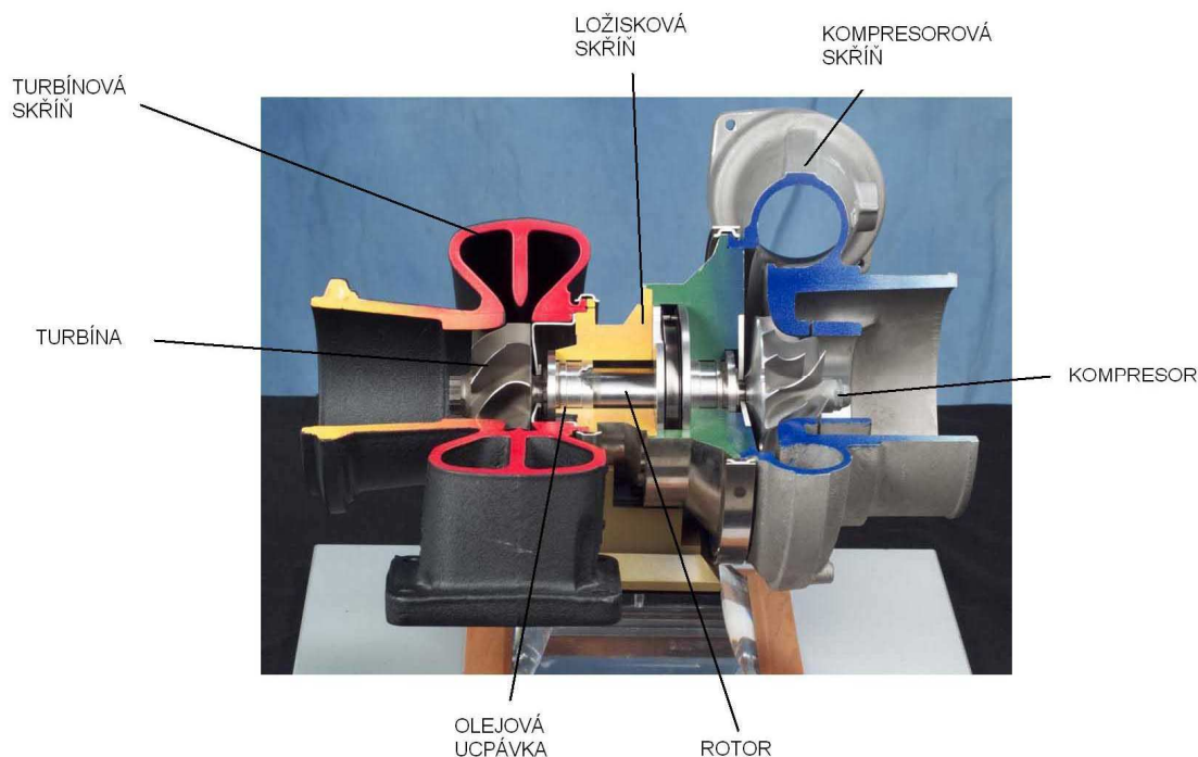
Obr. č. 2.1 – Základní části turbodmychadla[upraveno z 8]
