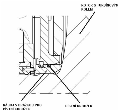
Obr.č. 5.6 – Turbínová ucpávka turbodmychadla NR20/S[upraveno z 12]
