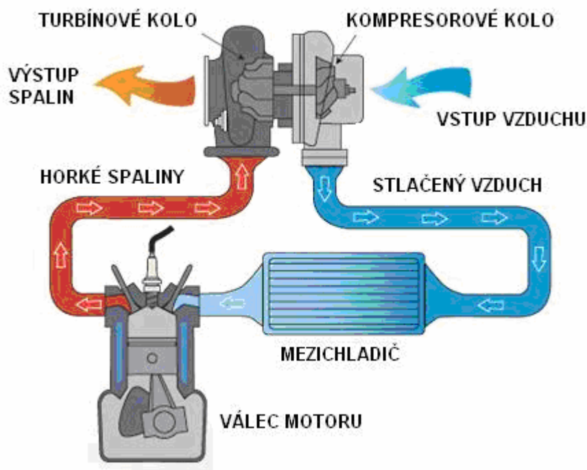
Obr.č.2.2 – Principiální schéma přepřňování spalovacího motoru[17]
