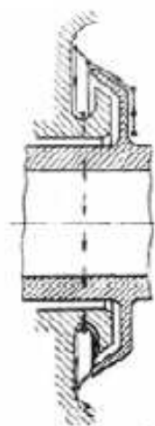
Obr.č.3.8 – Princip rozstříkovačích kroužku[5]
