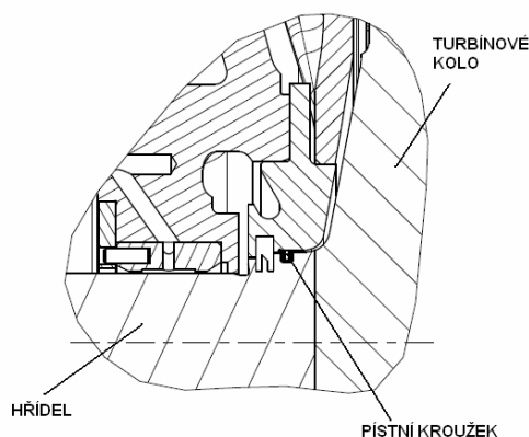
Obr.č. 5.7 – Turbínová ucpávka turbodmychadla TCR 14[upraveno z 12]
