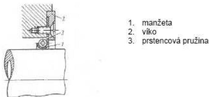
Obr.č. 3.10 – Manžetová ucpávka[5]
