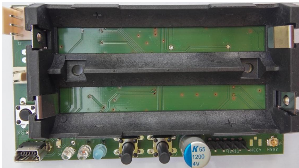
Osazená řídicí jednotka – horní strana
