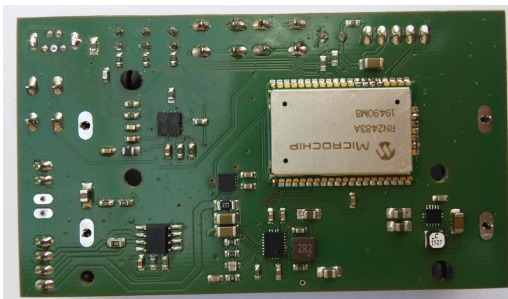
Osazená řídicí jednotka – spodní strana
