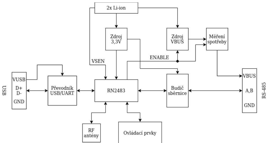
Obr. 23 - Blokové schéma elektroniky řídicí jednotky
