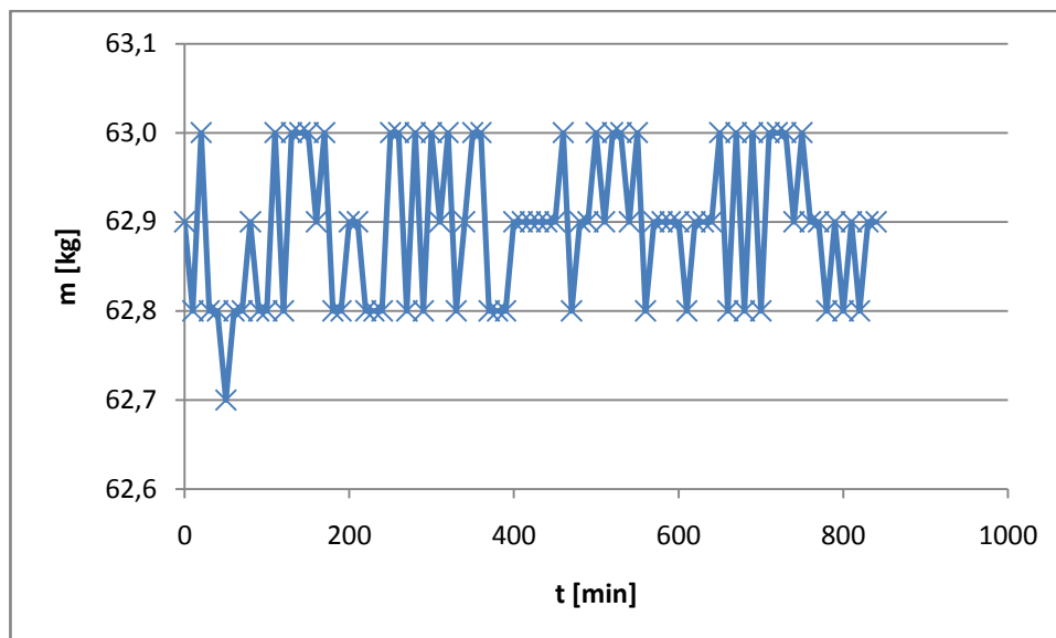
Obr. 39 - Závislost hmotnosti na čase s použitím tenzometru 1516084661
