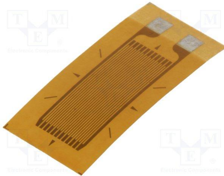
Obr. 9 - Kovový fóliový tenzometr [20]
