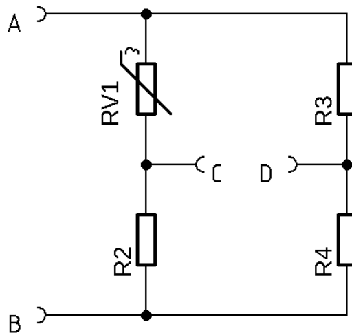
Obr. 10 - Schéma zapojení Wheatstoneova můstku s jedním tenzometrem
