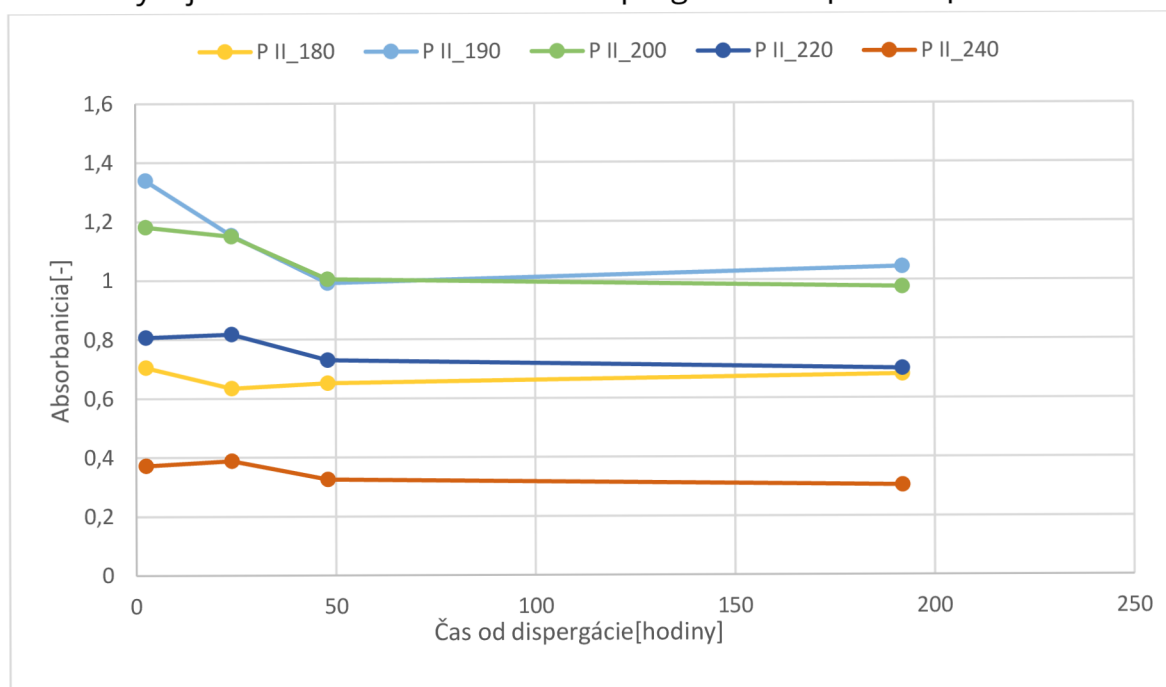
Graf 6: Vývoj absorbancií roztoku rGO dispergovaného plzmou pri atm. tlaku
