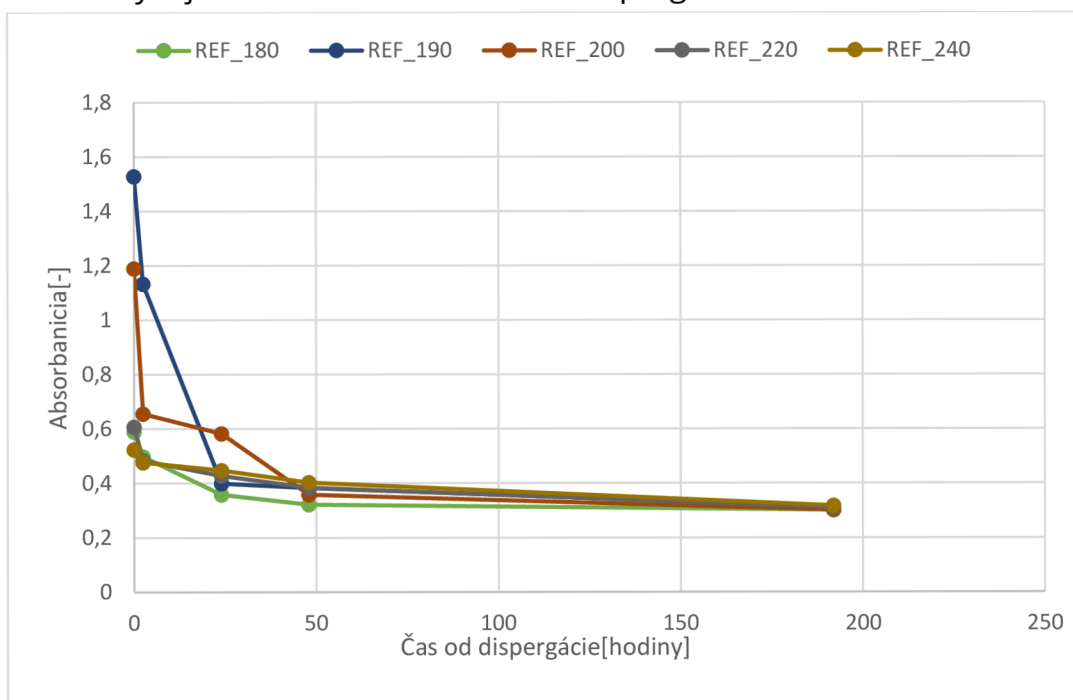
Graf 4: Vývoj absorbancií roztoku rGO dispergovaného referenčnou metódou
