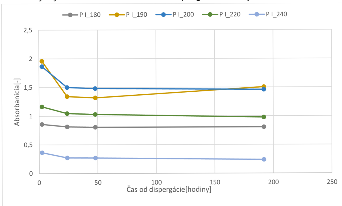
Graf 5: Vývoj absorbancií roztoku rGO dispergovaného hydrokavitáciou
