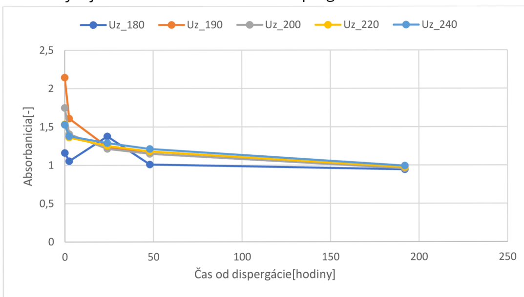
Graf 3: Vývoj absorbancií roztoku rGO dispergovaného sonikáciou
