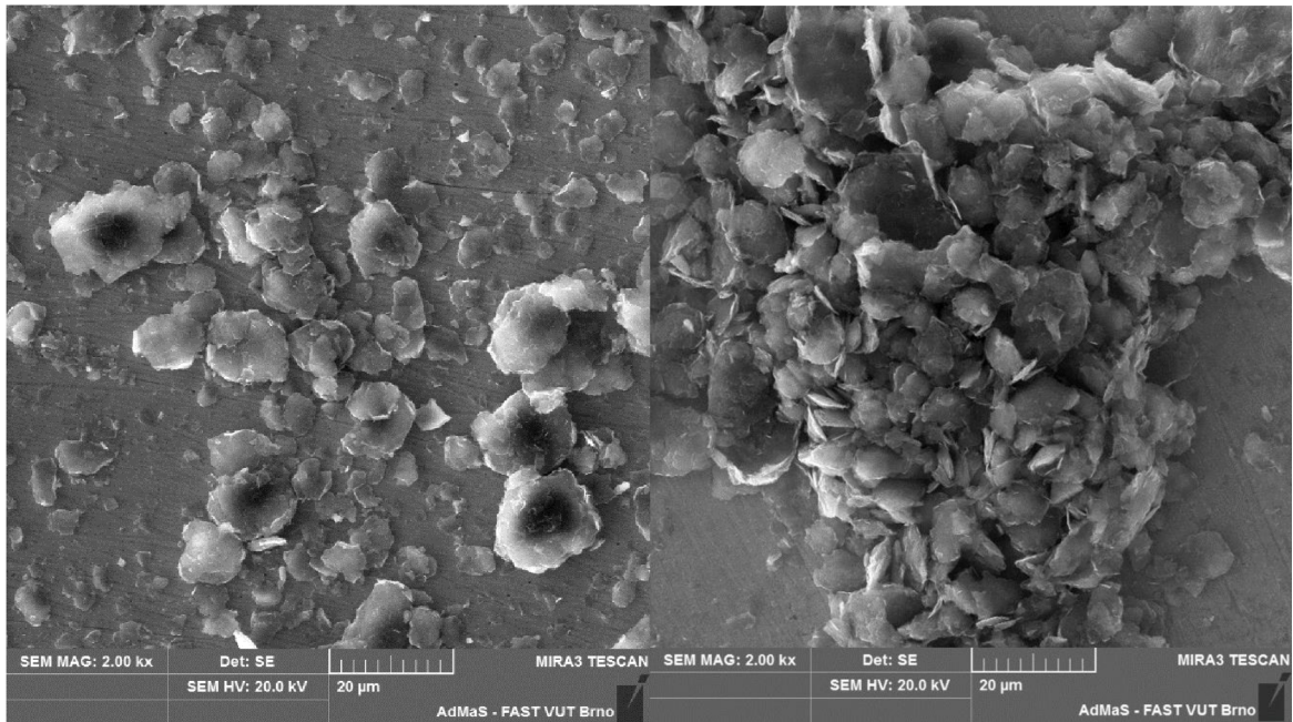
Obrázok 35: SEM snímky 2000x Uz – deň 0 a deň 7
