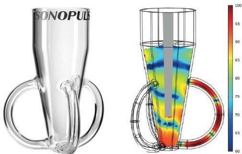
Obrázok 17: Rozetová nádoba Sonopuls a simulácia intenzity kavitácie v rozete [34]
