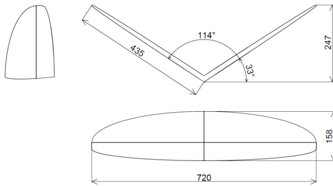
Obrázek 5-4 Základní rozměry ocasních ploch.
