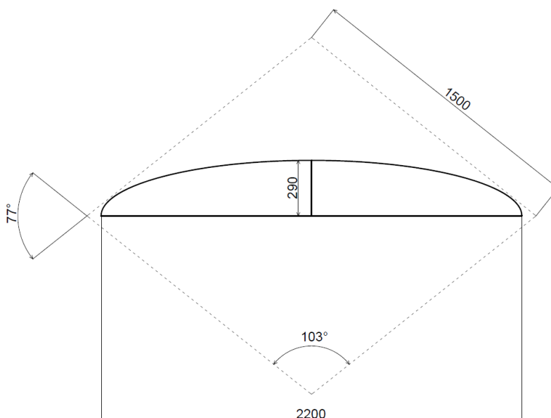
Obrázek 3-2 Druhá konfigurace [8].
