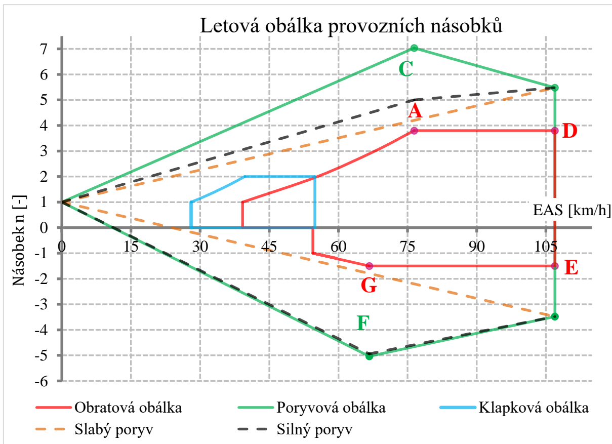
Obrázek 8-1 Letová obálka.
