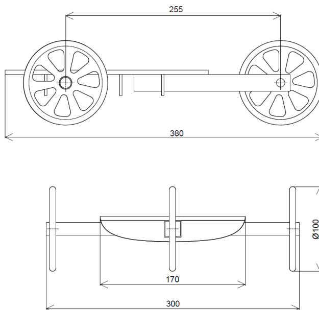
Obrázek 6-2 Výkres podvozku.
