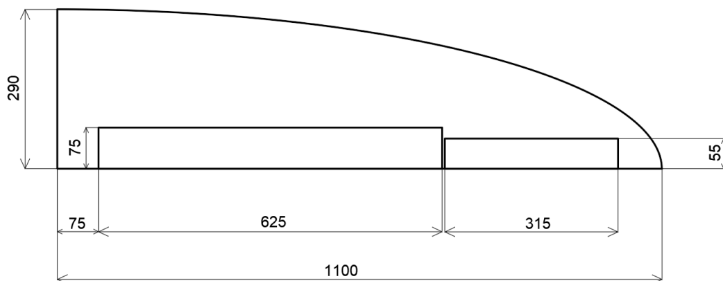
Obrázek 3-10 Vztlaková mechanizace [8].
