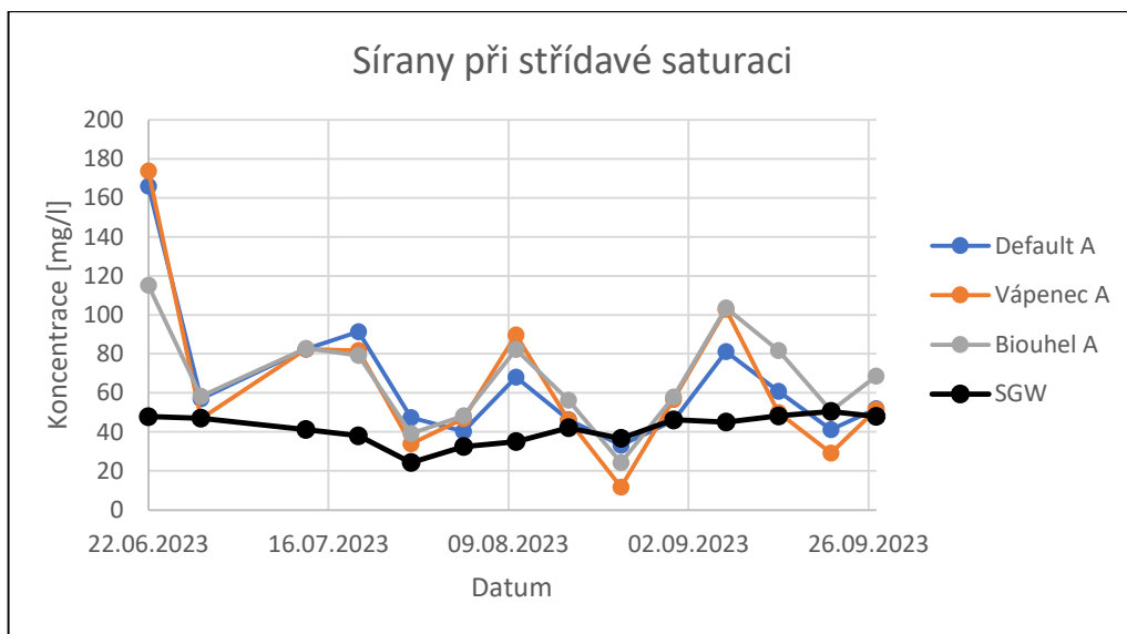
Graf 23: Naměřené hodnoty síranu u jednotlivých skupin střídavé saturace.
