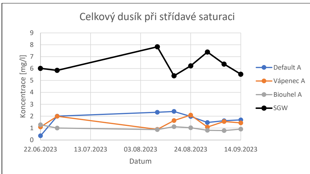
Graf 9: Koncentrace celkového dusíku při střídavé saturaci.
