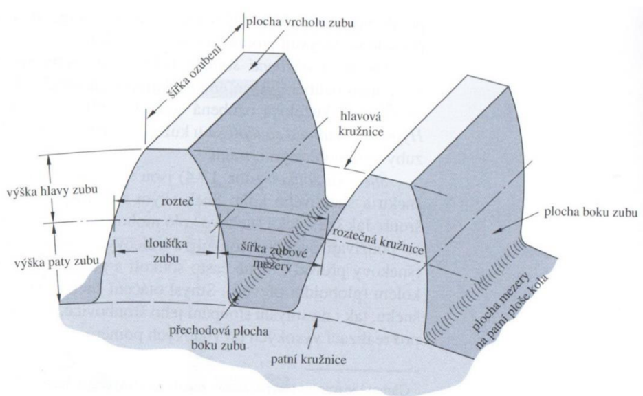
Obr. 21) Názvosloví ozubení [8]
