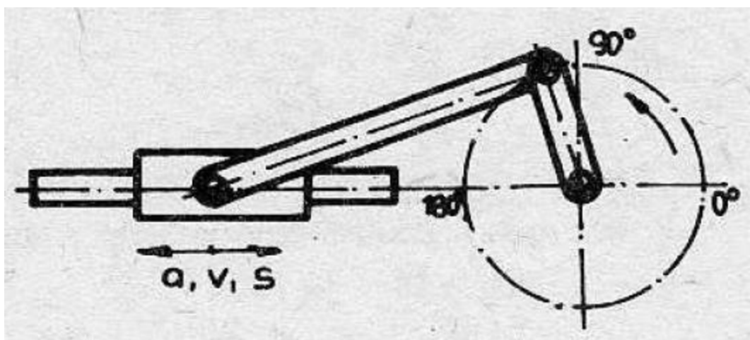
Obr. 5) Klikový mechanismus
