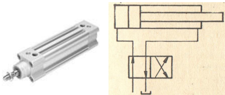
Obr. 9) Válec a píst a) příklad [10], b) ovládání [7]
