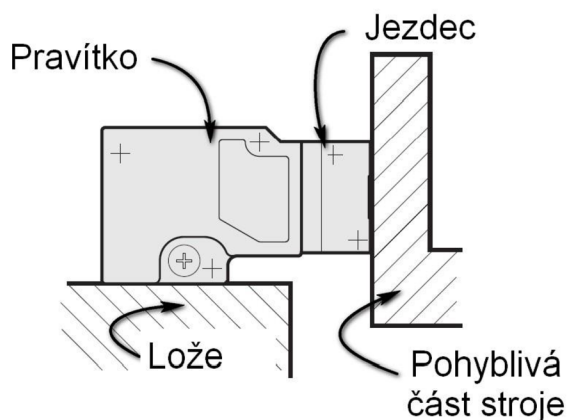
Obr. 54) Uložení pravítka
