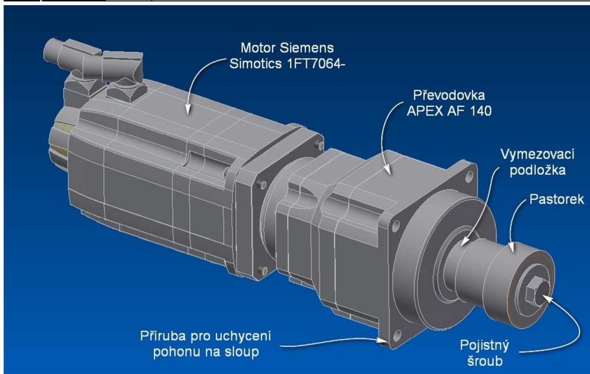
Obr. 50) Sestava pohonu
