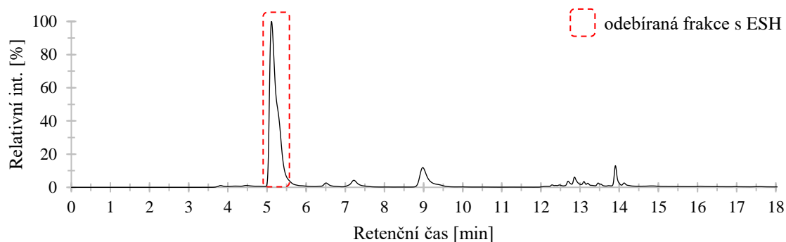
Obr. 7: Preparativní HPLC
