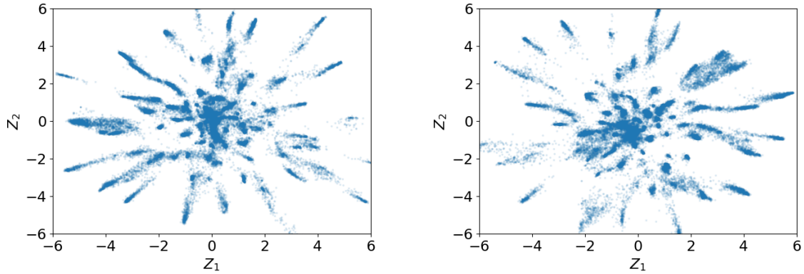
Obrázek 8.2: Latentní prostor pro query sekvenci PIP_BREBN/26-275 s ponecháními mezerami ( vlevo ) a bez mezer ponechaných mezer mimo pozice query sekvence ( vpravo ).
