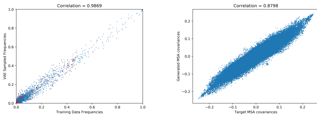
Obrázek 8.11: Statistika prvního a druhého řádu pro konečný model s jednou skrytou vrstvou s 450 neurony vybraného pro experiment. Vlevo: statistika prvního řádu s vysokou korelací značí schopnost VAEs reflektovat frekvence aminokyselin na daných pozicích. Vpravo: korelace kovariance statistik druhého řádu.
