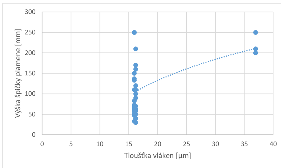
Graf 10: Závislost výšky špičky plamene na tloušťce vláken
