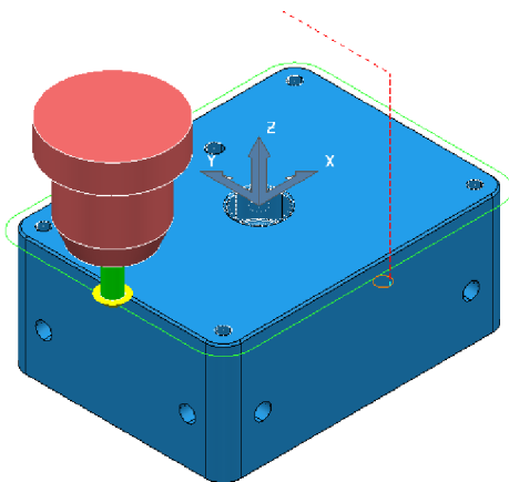
Obr. 34 Sražení obvodové hrany.
