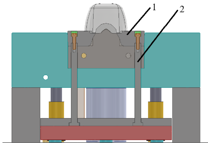
Obr. 13 Stírací deska.
