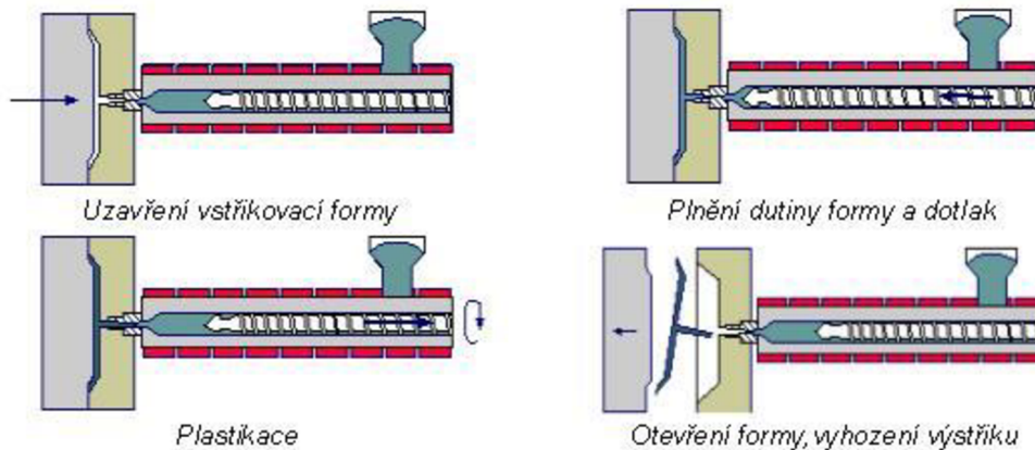
Obr. 5 Průběh vstříkování [11].
