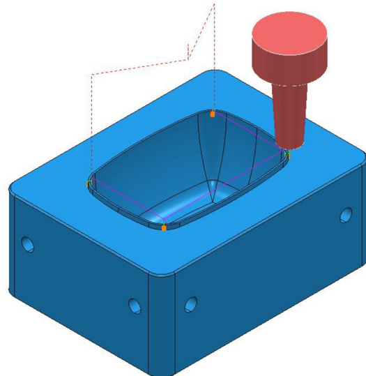
Obr. 50 Frézování drážek.
