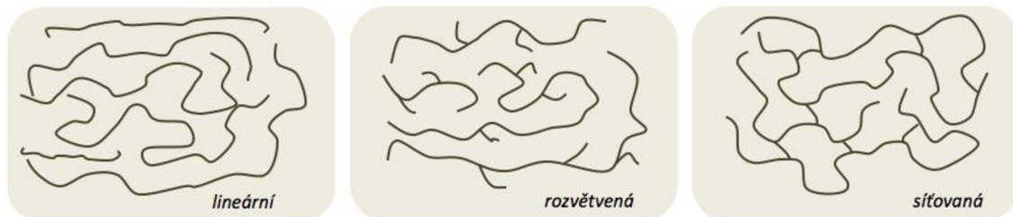
Obr. 3 Tvar makromolekul [1].
