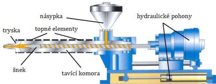
Obr. 8 Schéma vstříkovací jednotky [12].
