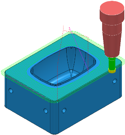
Obr. 47 Dokončení čela.
