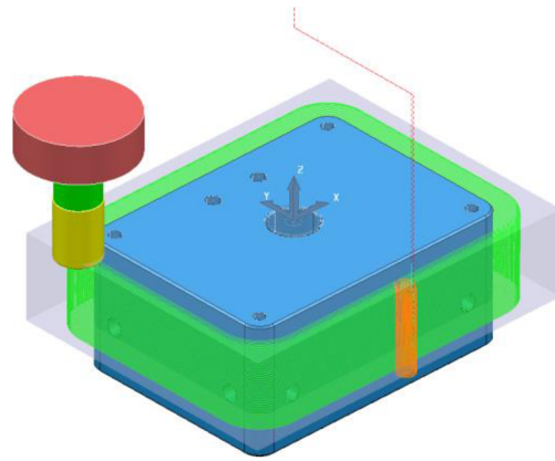
Obr. 25 Hrubování obvodu.
