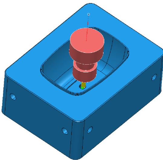
Obr. 55 Dohrubování otvoru trysky.
