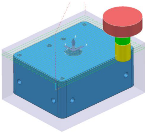
Obr. 24 Hrubování čela.
