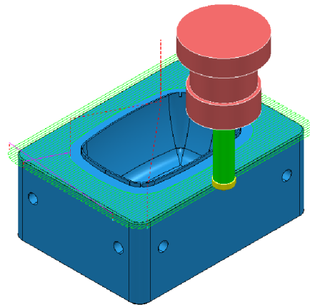
Obr. 43 Dohrubování čela.
