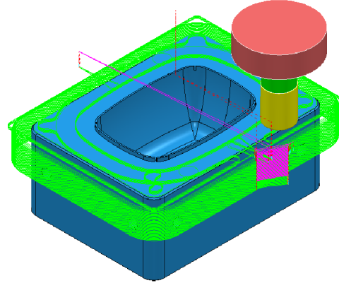
Obr. 37 Hrubování obvodu.
