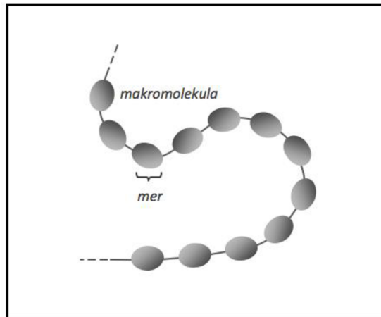
Obr. 2 Makromolekula [1].
