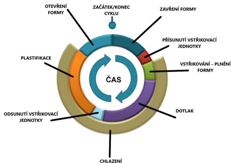
Obr. 6 Cyklus vstřikování [13].
