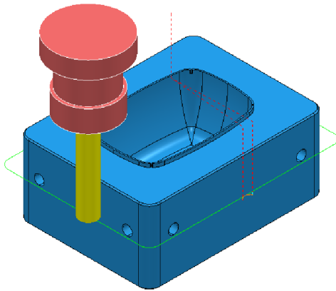
Obr. 42 Dohrubování obvodu.
