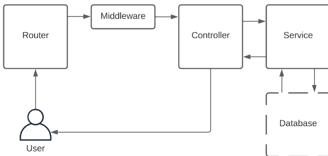
Obr. 6 Životní cyklus požadavku
