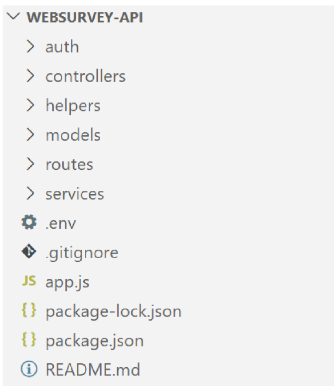
Obr. 5 Struktura backendu
