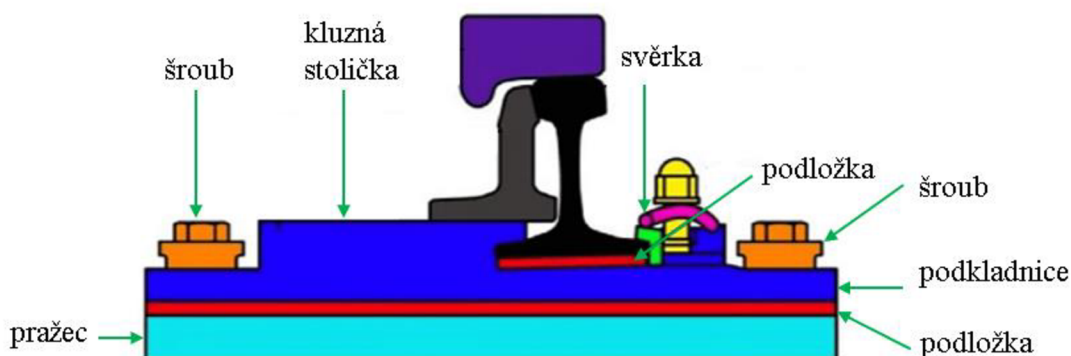
Obrázek 8: Nepřímé upevnění kolejnice výhybky [25]
