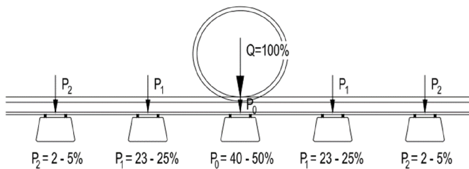
Obrázek 6: Rozdělení kolové síly na jednotlivé pražce [20]
