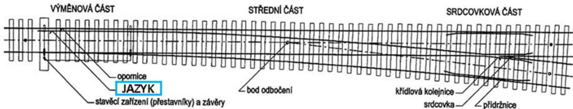
Obrázek 1: Schéma výhybky s jazykem [4]
