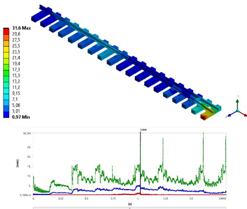
Obrázek 37: Celková deformace modelu v čase (zeleně maximální), přejezd 40 \frac{km}{h}
