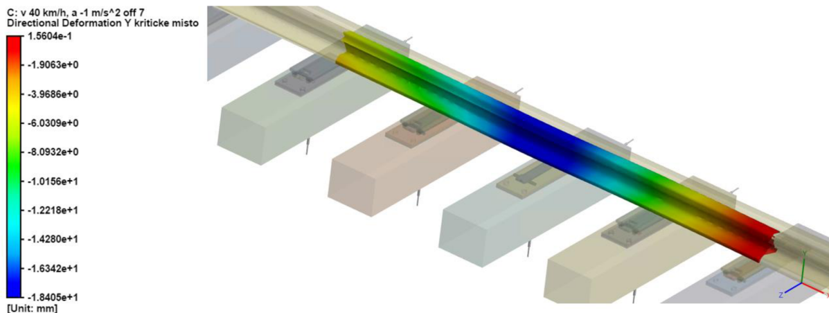
Obrázek 49: Y deformace s maximem v místě chybějící 7. stoličky
