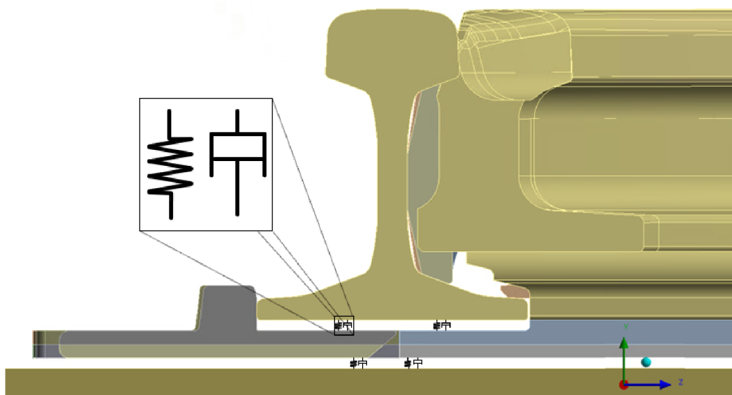
Obrázek 22: Nastavení vazeb podložek
