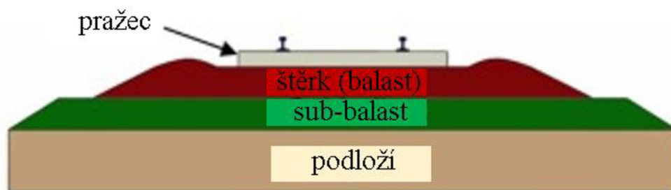
Obrázek 3: Klasická konstrukce trati (převzato a upraveno z [11])
