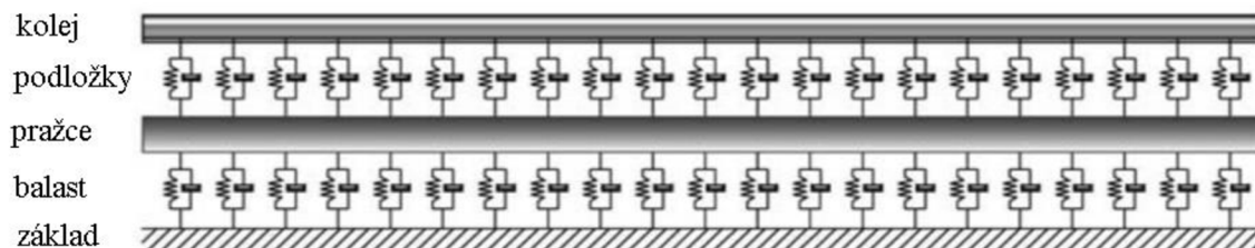
Obrázek 11: Dvouvrstvý spojitý model tratě (převzato a upraveno z [17])
