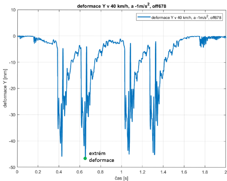
Obrázek 52: Průběh Y deformace v čase při ztrátě podpory jazyka 6., 7. a 8. stoličkou
