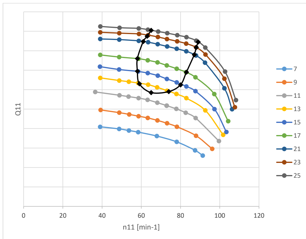
Graf 3 Vykreslení křivky účinnosti 80 %
