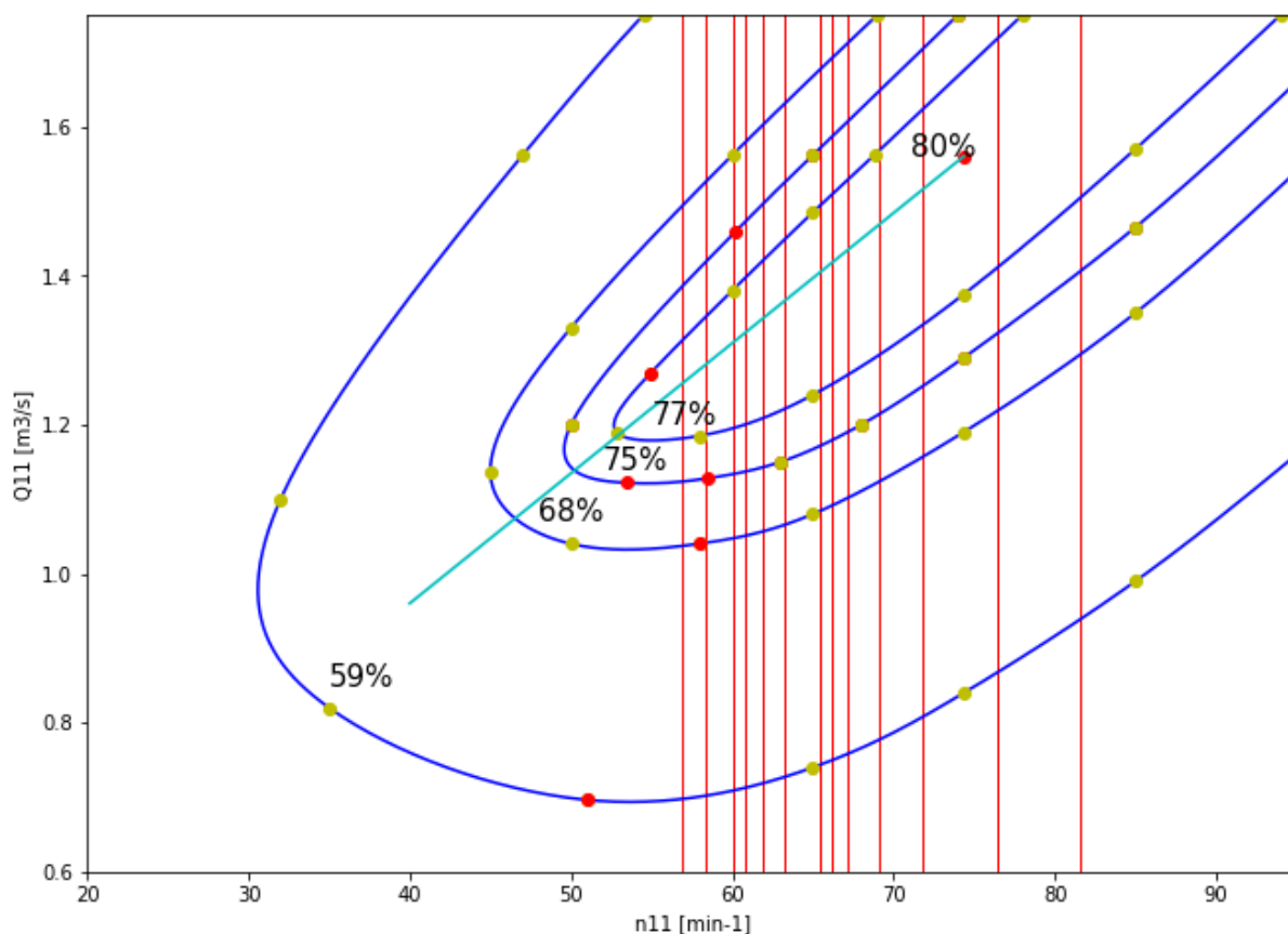
Graf 16 Charakteristika menší turbíny D=1,56 m
