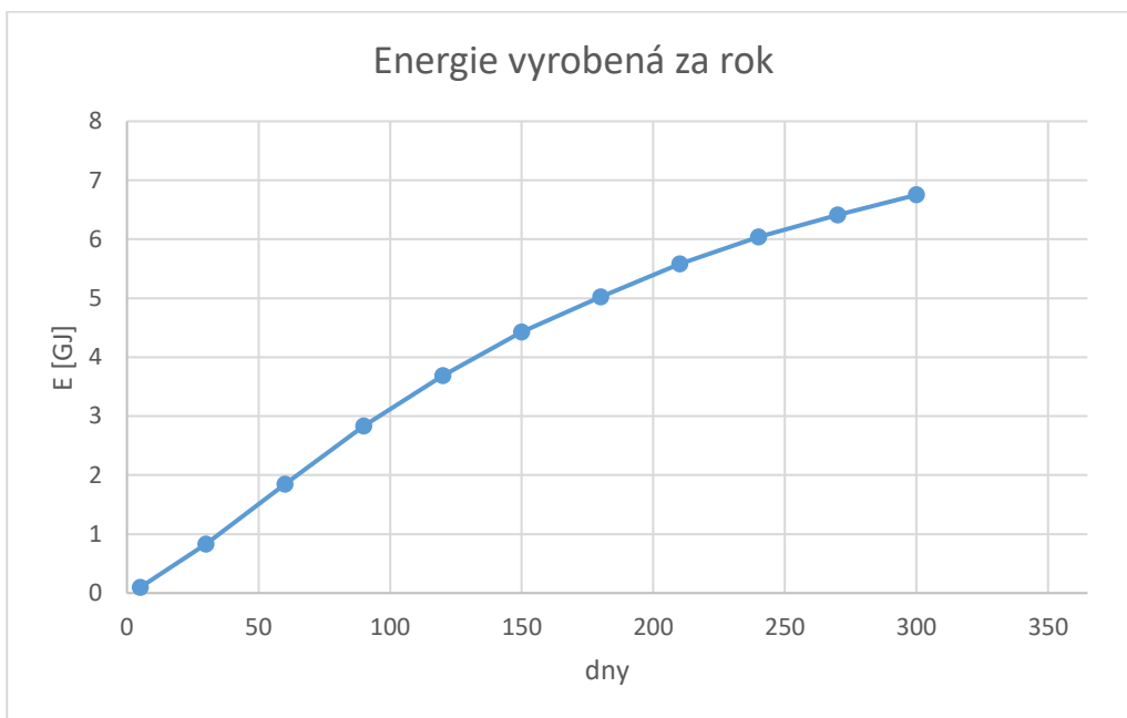
Graf 18 Vyrobená energie za rok v GJ
