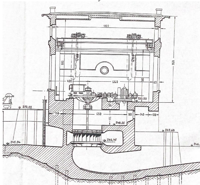
Obr. 13 Příčný řez elektrárnou
