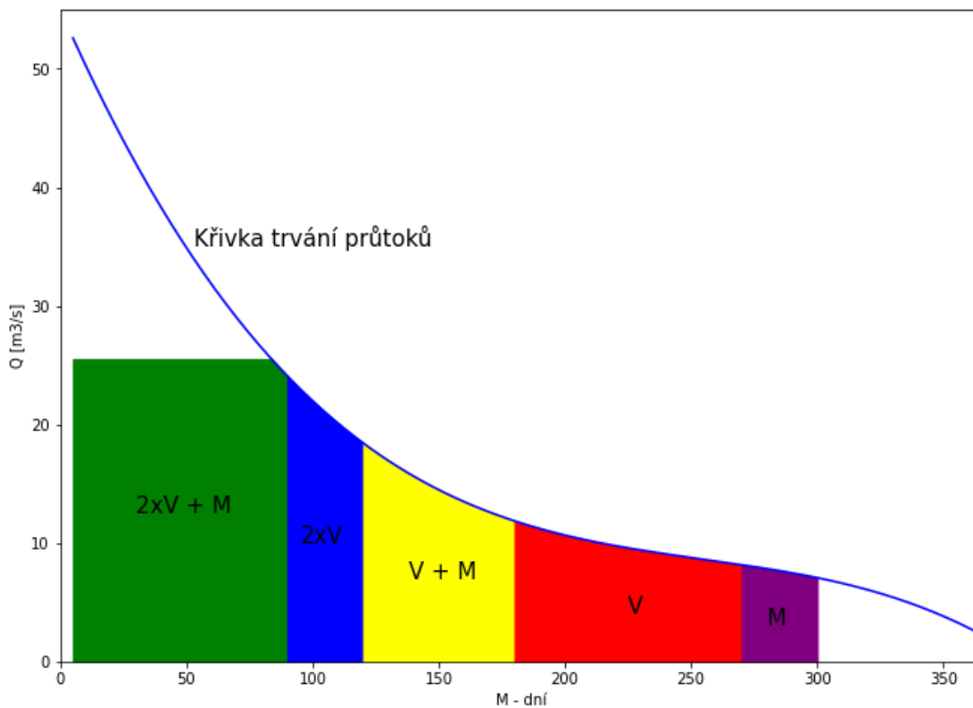
Graf 19 Znáornění využití potenciálu elektrárnou s vyznačením provozu jednotlivých turbín
