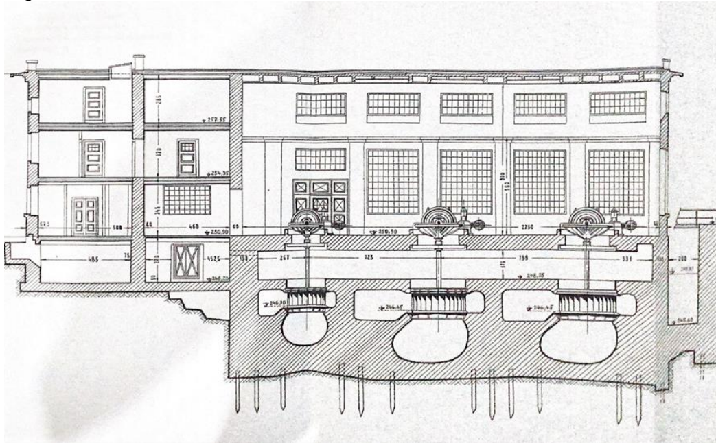
Obr. 12 Podélný řez elektrárnou
