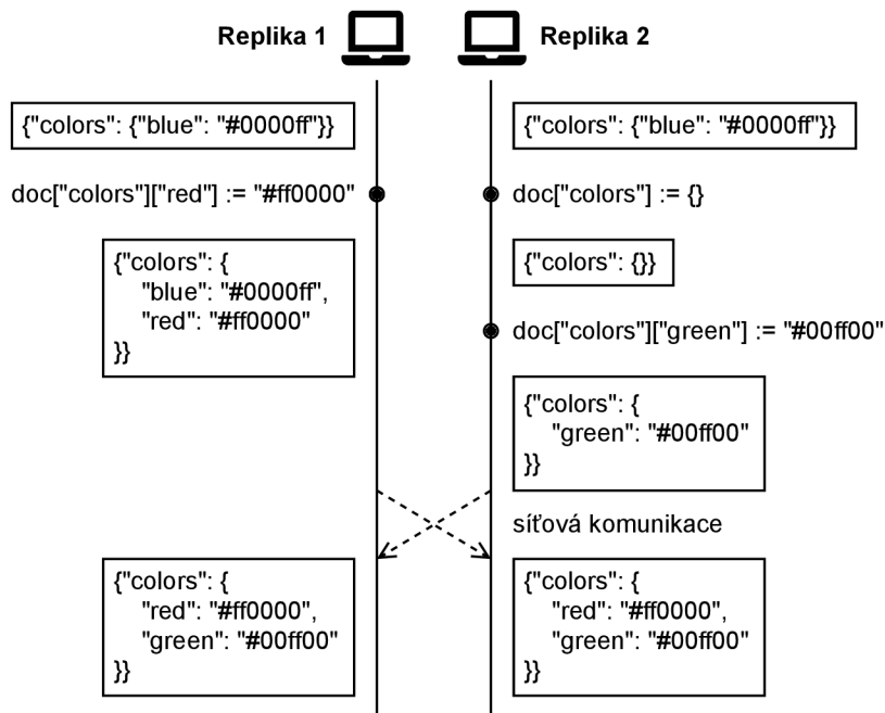
Obrázek 3.3: Úpravování obsahu zanořenému objektu map a souběžné přepsání celého objektu map. Zdroj [27].
