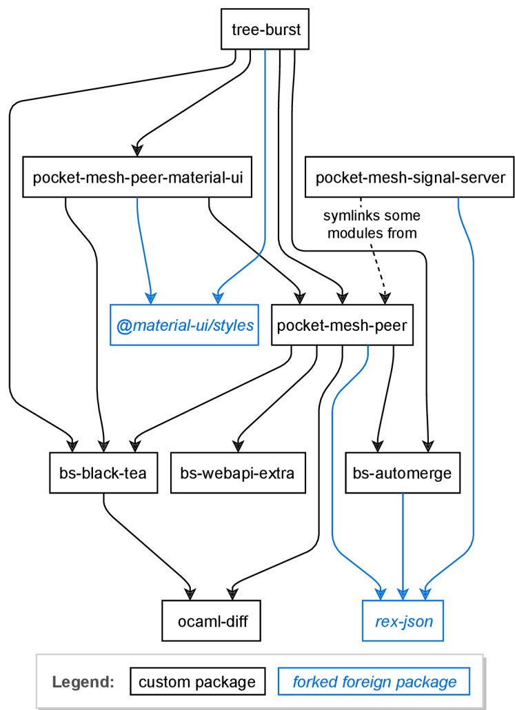
Obrázek 4.1: Graf závislostí balíčků (podprojektů).
