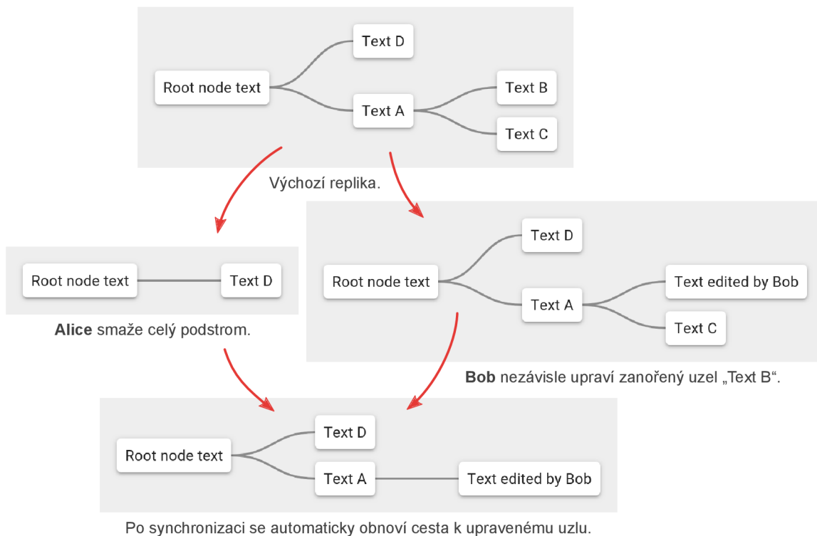
Obrázek 6.3: Automatické aplikačně-specifické řešení konfliktu.
