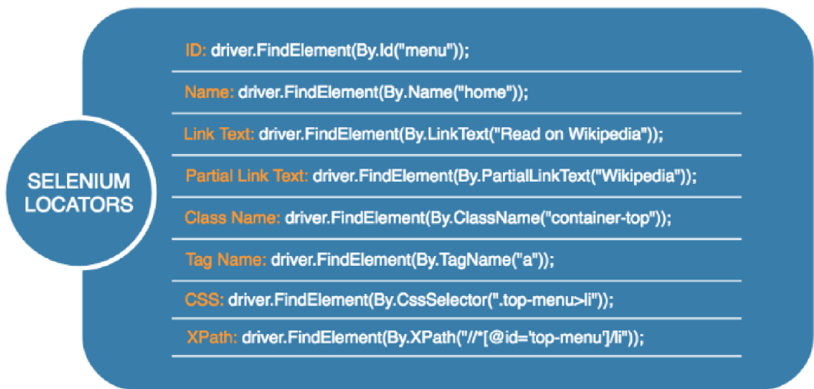
Obrázek 8: Selenium Lokátory
