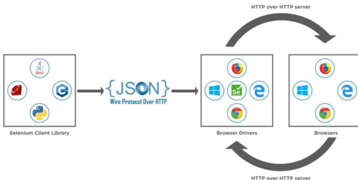
Obrázek 6: WebDriver Architecture
