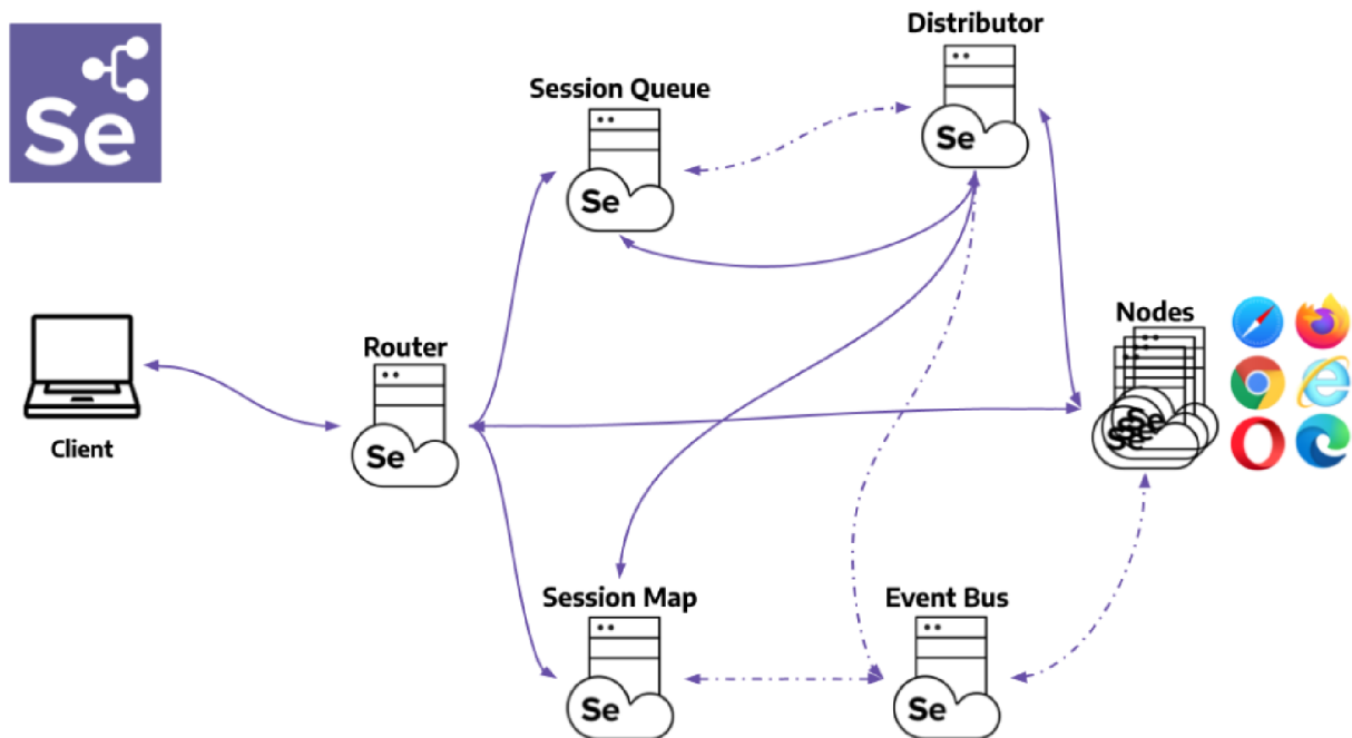
Obrázek 7: Selenium Grid
