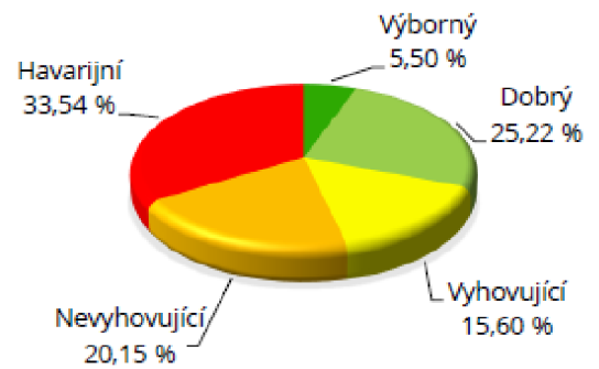
Graf 34: Stav povrchu vozovek okres Jablonec n. Nisou 2017
