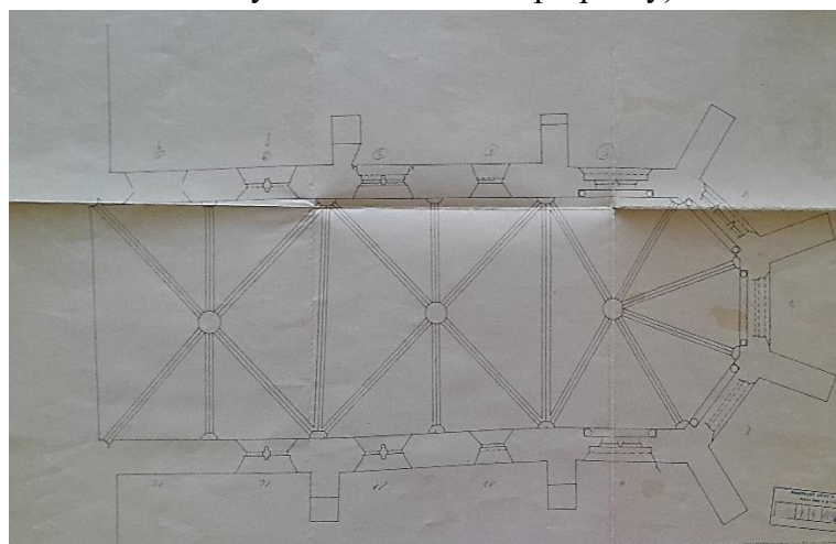
18. Jihlava, půdorys presbytáře kostela Povýšení sv. Kříže
