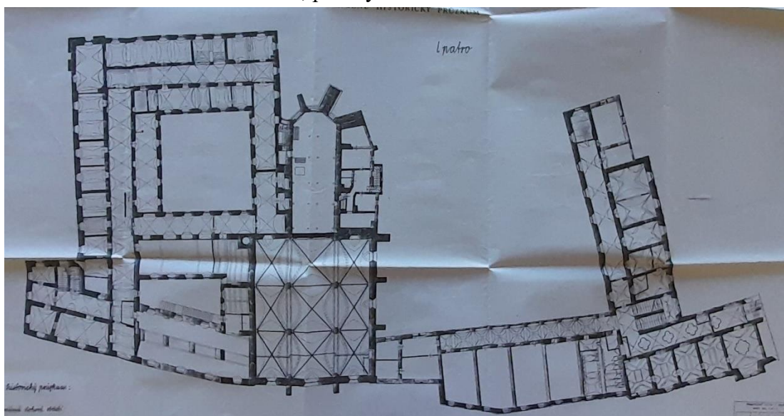
17. Jihlava, půdorys kláštera a kostela Povýšení sv. Kříže (ještě před úpravami a vybouráním chórové přepážky)
