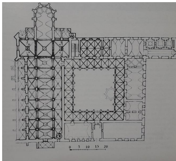
77. Zlatá Koruna, klášter, půdorys
