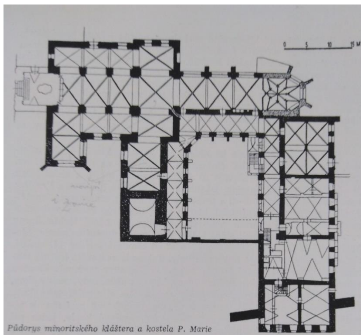
14. Jihlava, půdorys kláštera a kostela Nanebevzetí Panny Marie
