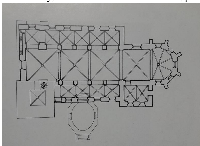
143. Písek, kostel Panny Marie, půdorys
