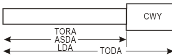
Obr. 3: RWY vybavena CWY, Zdroj: předpis L14
