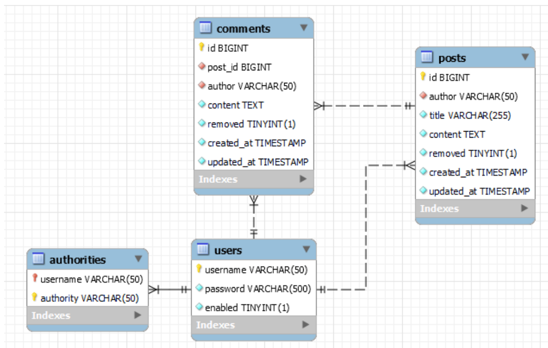
Obrázek 1: ERD Diagram
