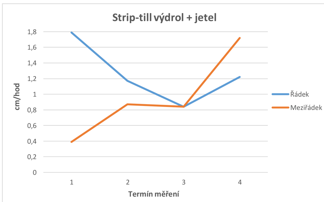
Graf 7: Vývoj nenasyčené hydraulické vodivosti u pásového zpracování půdy s meziplodinou výdrolu pšenice a jetele
