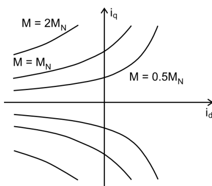
Obrázek 2.11: Trajektorie konstantního točivého momentu [17]
