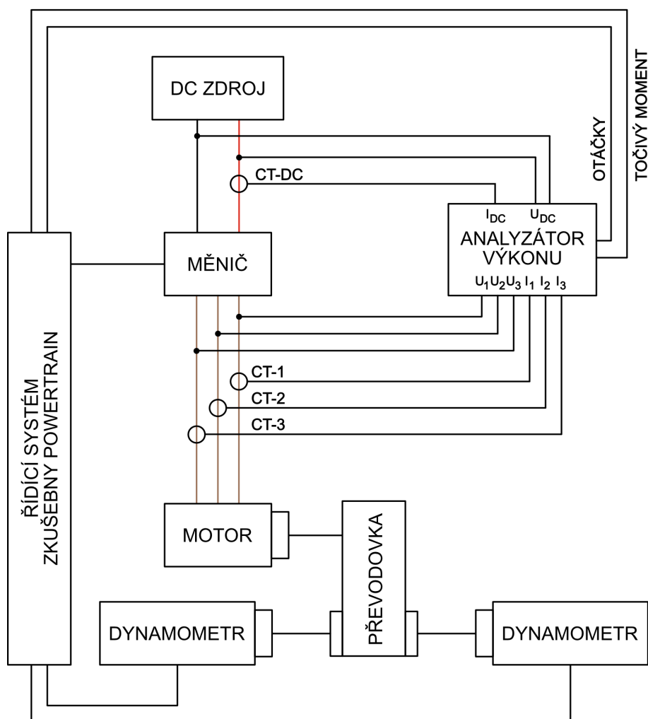
Obrázek 10.3: Schéma experimentu měření účinnosti hnacího ústrojí
