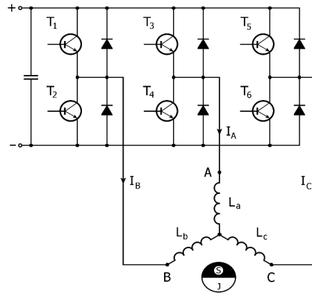
Obrázek 2.4: Elektrické zapojení střídače [30]
