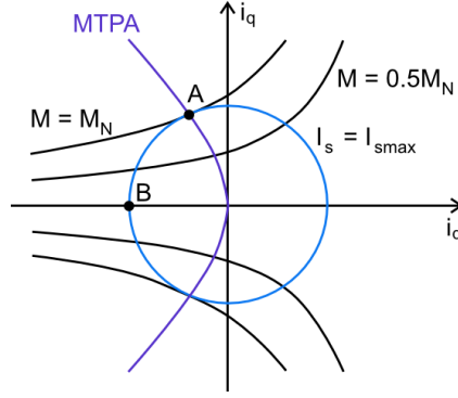
Obrázek 2.12: Trajektorie metody řízení MTPA [20]
