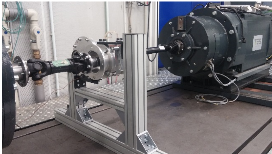
Obrázek 9.3: Umístění převodovky ve zkušebně powertrain
