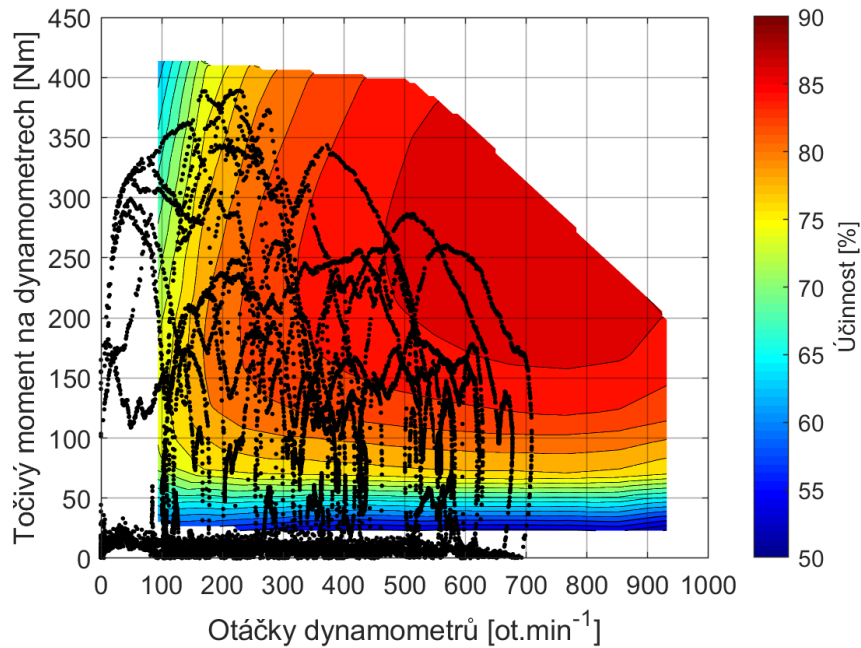
Obrázek 10.11: Body provozu hnacího ústrojí při jízdním cyklu WLTC Class 2 v celkové mapě účinnosti hnacího ústrojí
