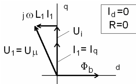
Obrázek 2.10: Fázorový diagram řízení PMSM na maximální točivý moment [30]
