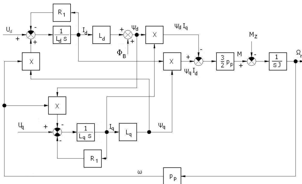
Obrázek 2.7: Blokové schéma modelu PMSM [30]
