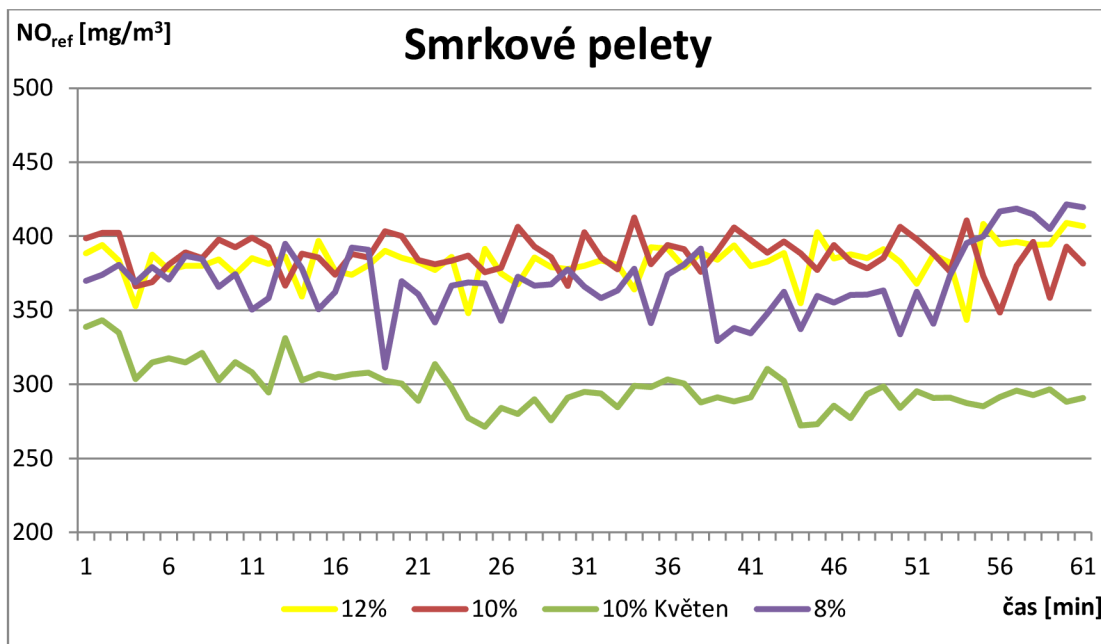
Obr. 7-16 Graf referenčních hodnot NO pro smrkové pelety
