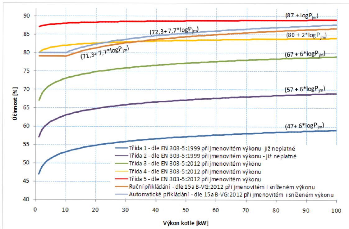
Obr. 7-27 Graf určující emisní třídu kotle[29]
