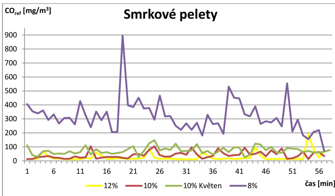
Obr. 7-17 Graf referenčních hodnot CO pro smrkové pelety
