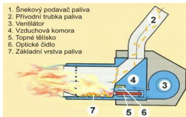
Obr. 4-7 Trubicový hořák[18]
