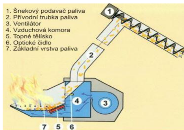
Obr. 4-5 Miskový hořák[18]
