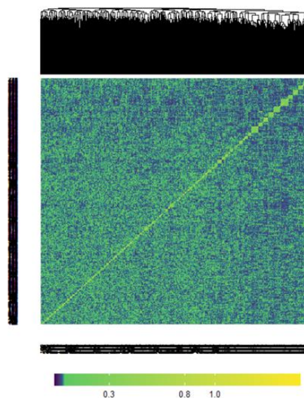
Obrázek 1- genetická matice sledovaných jedinců zobrazující vzájemnou realizovanou příbuznost testovaných semenáčků.
