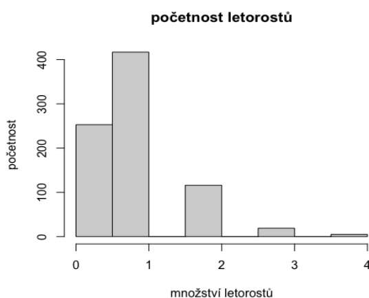
graf 4-histogram početnosti počtu letorostů
