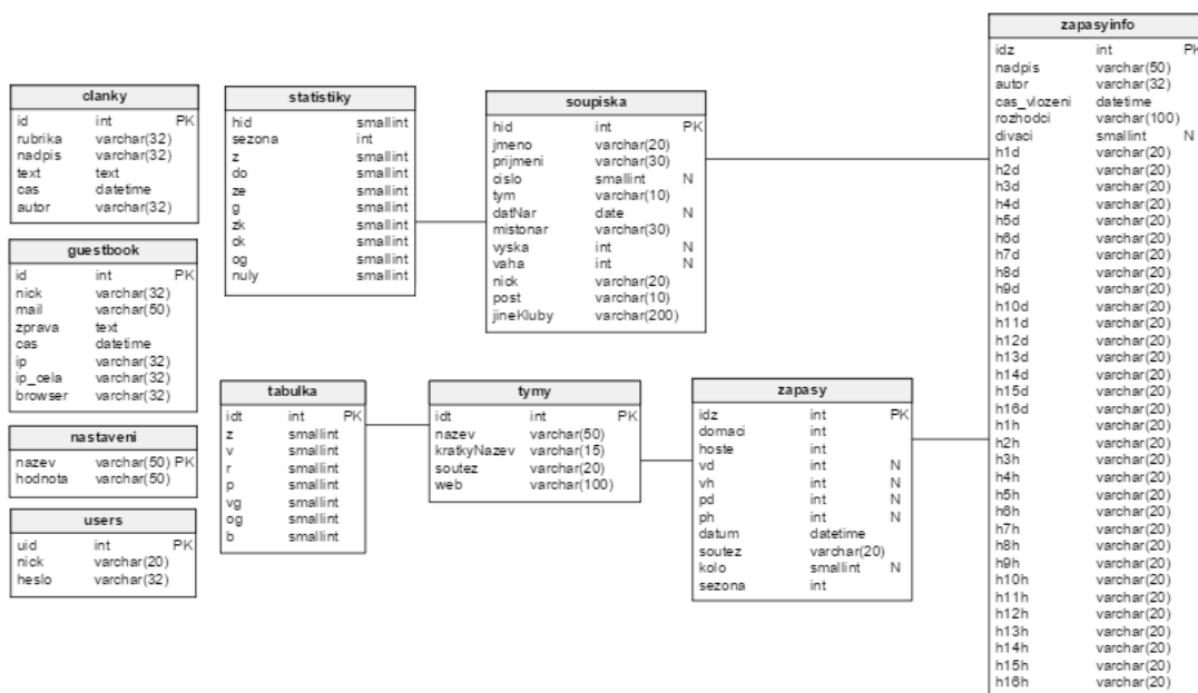
Obrázek 1: Schéma databáze (zdroj: aplikace dostupná na http://www.vertabelo.com )
