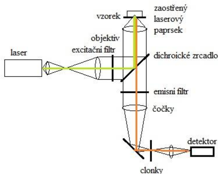
Obr. č. 10: Schéma konfokálního mikroskopu. Excitační laserové světlo (naznačeno zelenou barvou) je vedeno do objektivu, kde je fokusováno do vzorku a odraženo zpět, dále prochází přes dichroické zrcadlo a emisní filtr do detektoru.
