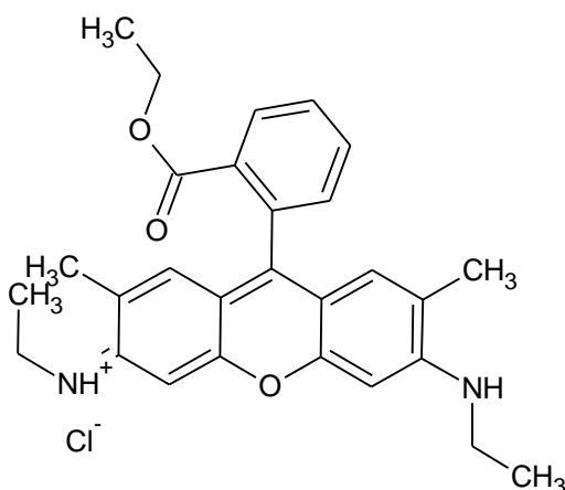
Obr. č. 8: Struktura Rhodaminu 6G
