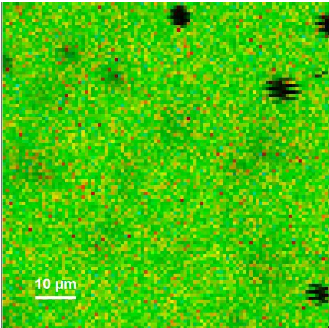
Obr. č. 13: FLIM analýza fluoresceinu v gelu
