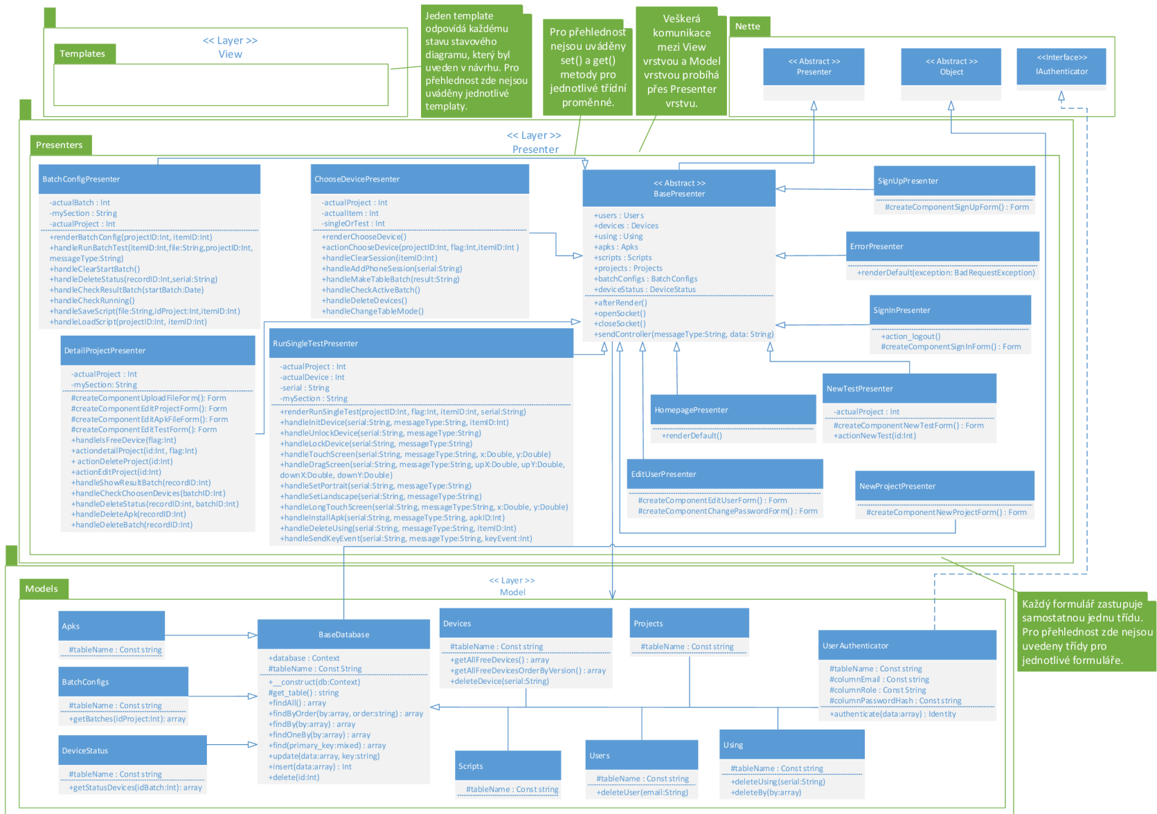
Obrázek B.1: Diagram tříd uživatelského modulu.
