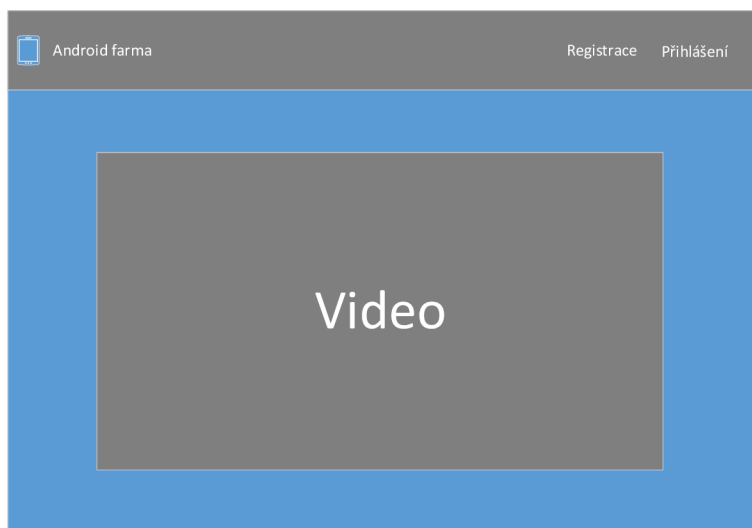
Obrázek 4.8: Úvodní okno.
