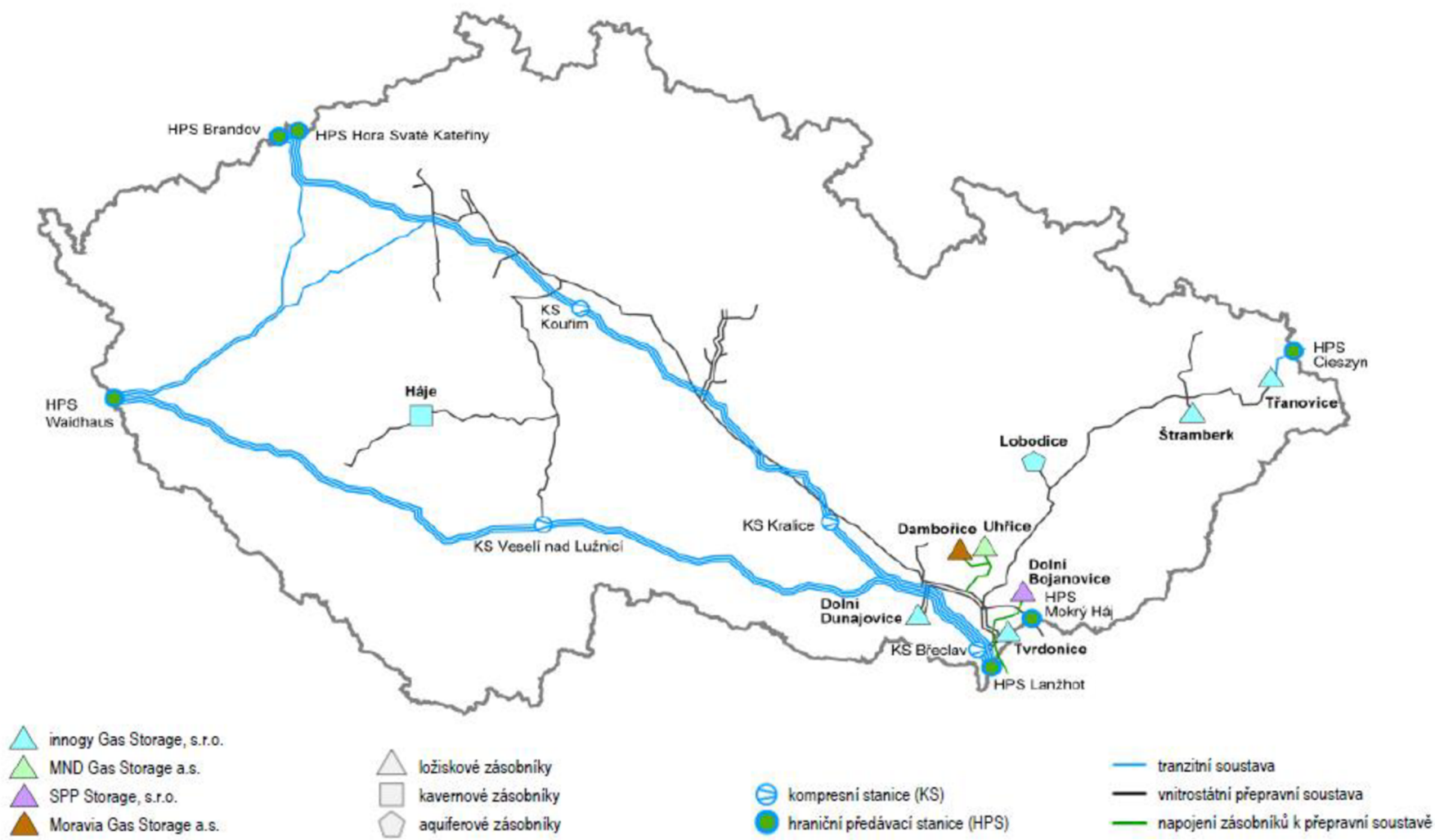
Obr. 2.4 Schéma přepravní soustavy a zásobníků plynu v ČR [25]
