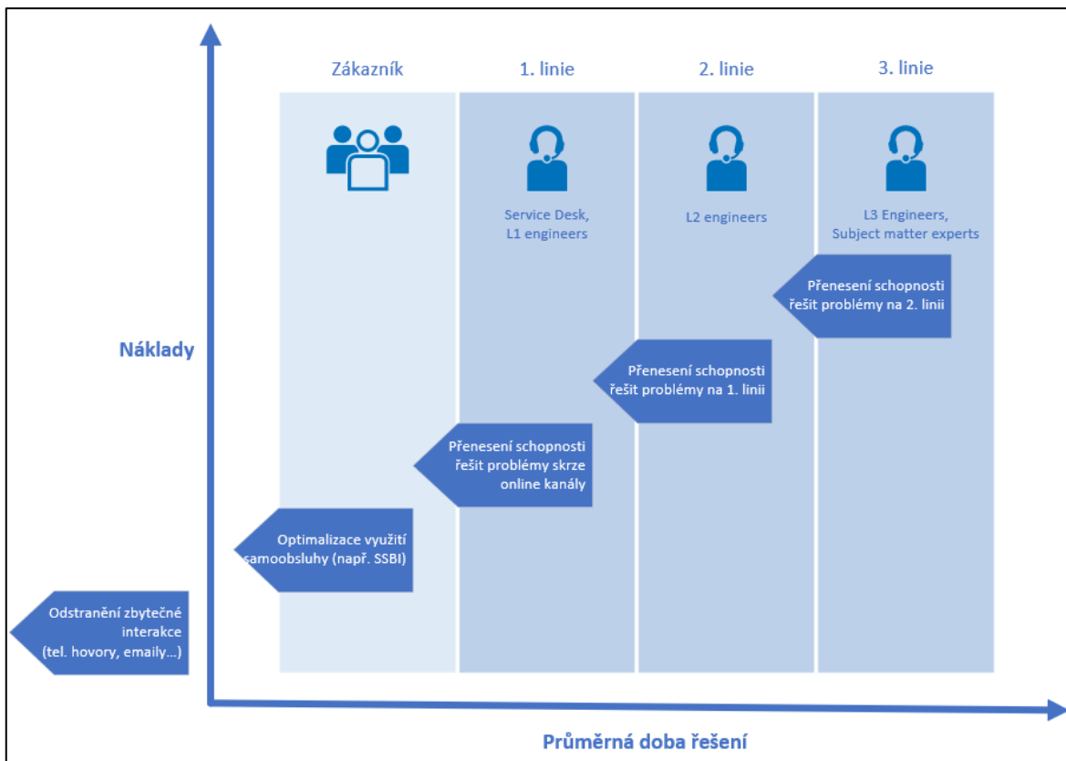
Obrázek 22- Shift-Left vizualiace 39
