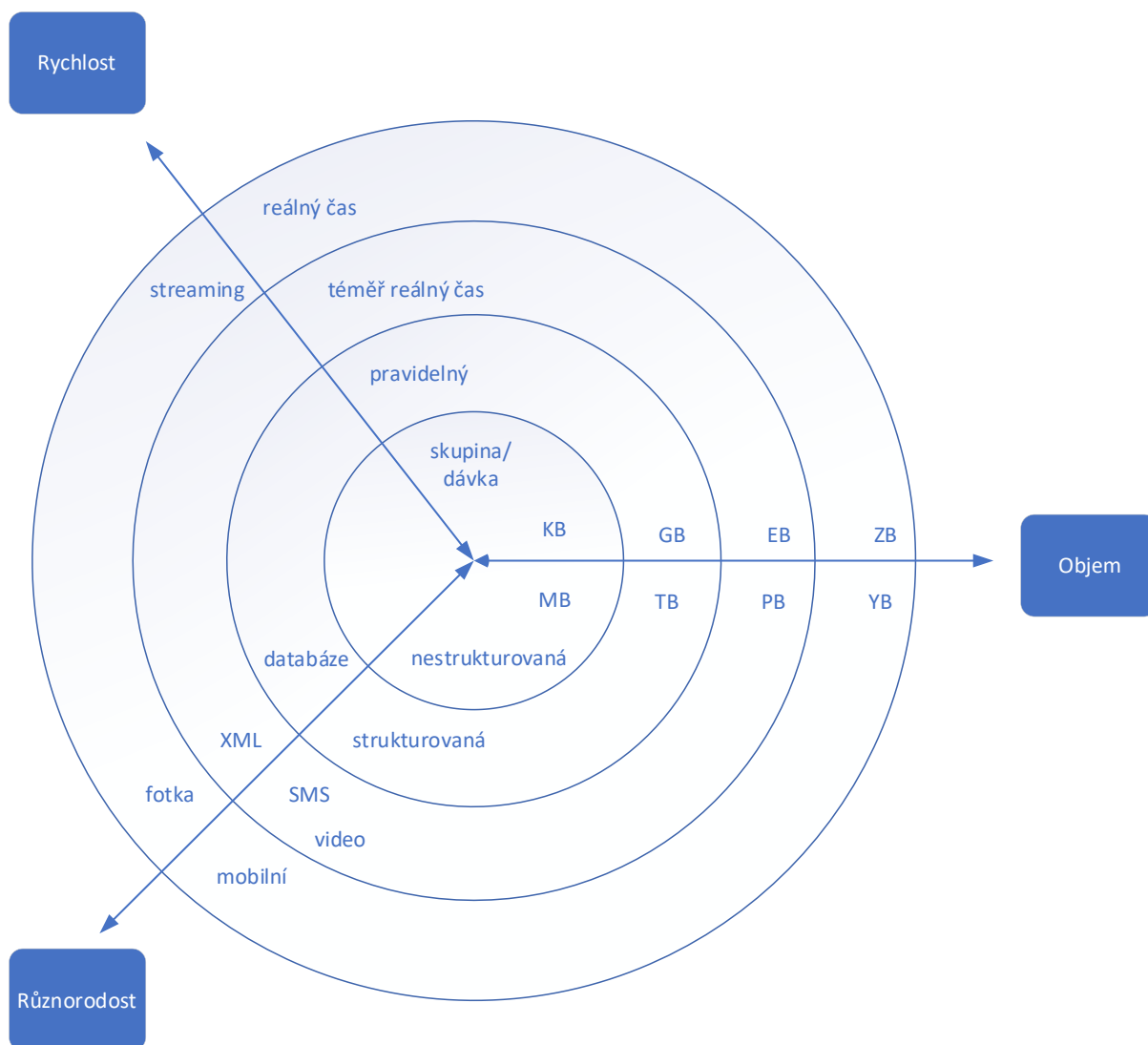
Obrázek 11- Model 3V 19
