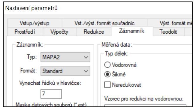
Obrázok 19 – Nastavenie parametrov
