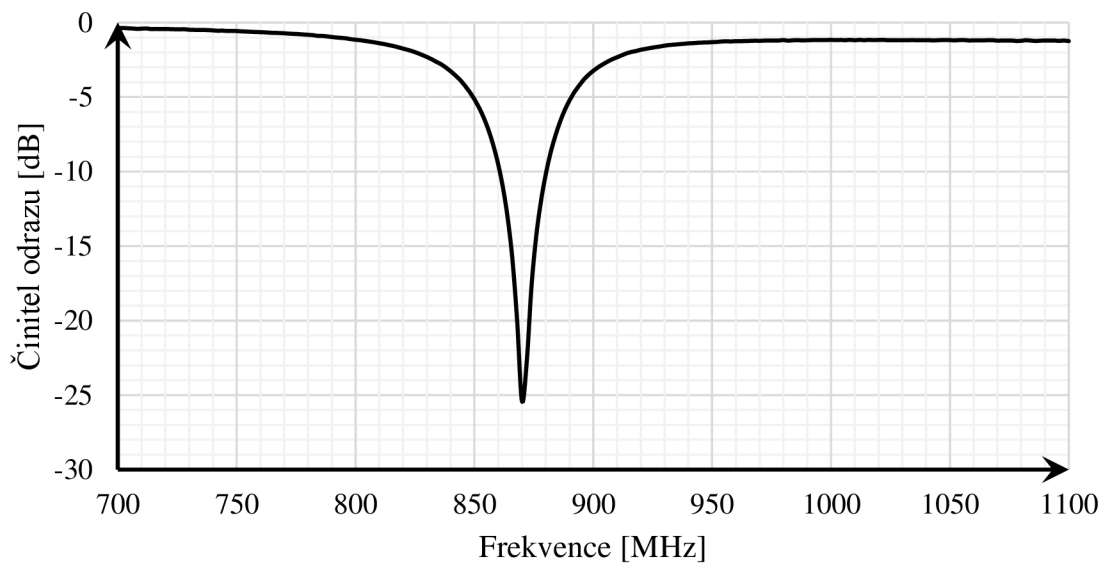
Obr. 4.12: Činitel odrazu impedančně přizpůsobené čipové antény
