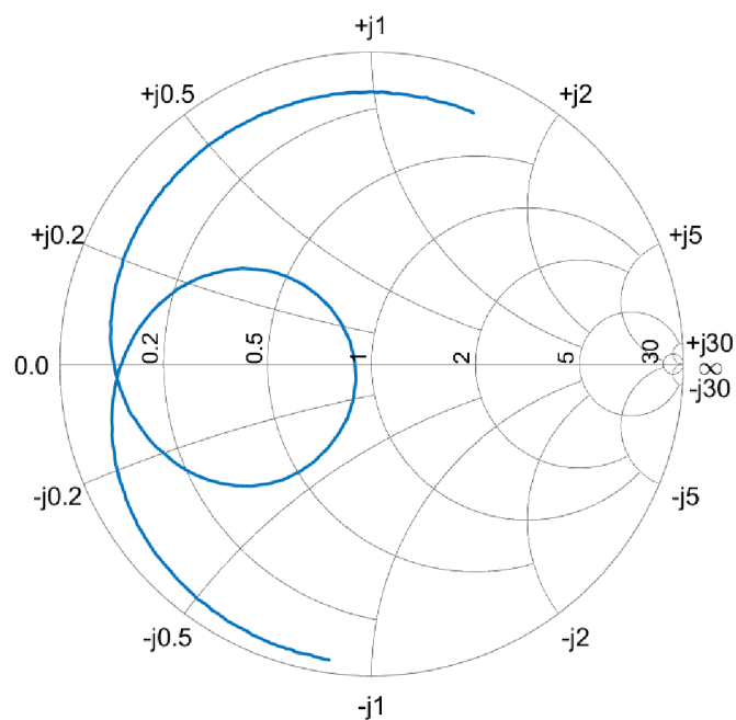
Obr. 4.13: Impedance impedančně přizpůsobené čipové antény (Smithův diagram)
