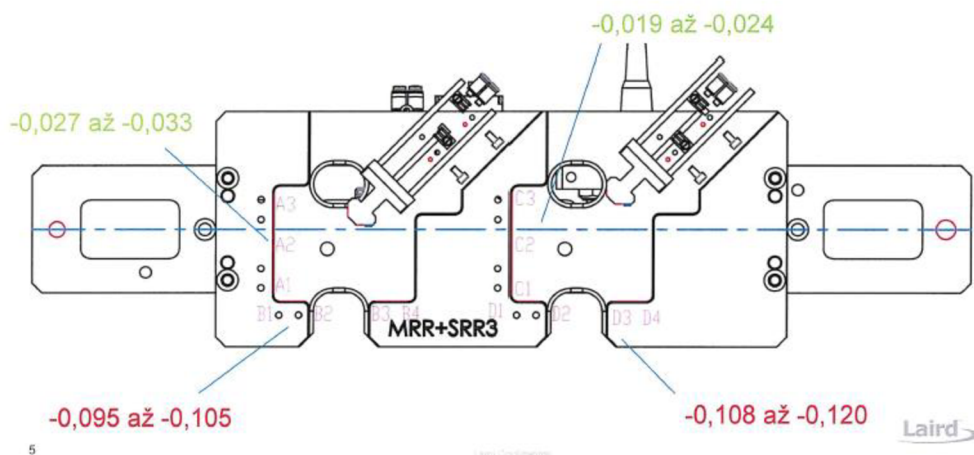
Obrázek 29: Návrh lůžek
