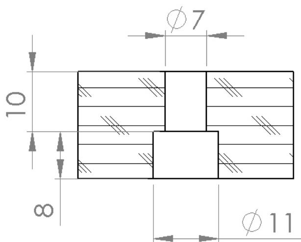
Obrázek 3.16: Řez dírou pro šroub na základně extrudéru
