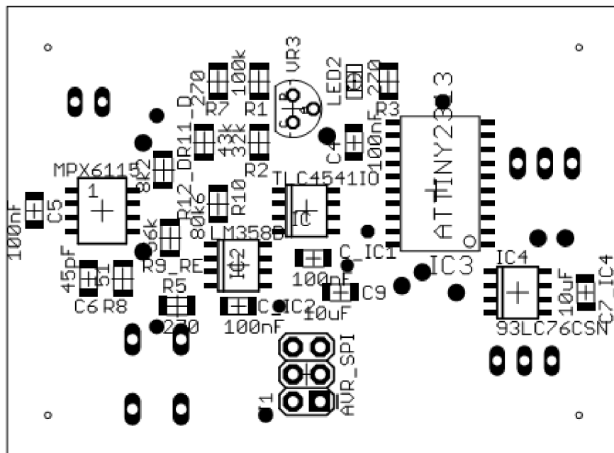
Rozměr desky 35 x 22 [mm], měřítko M1:2
