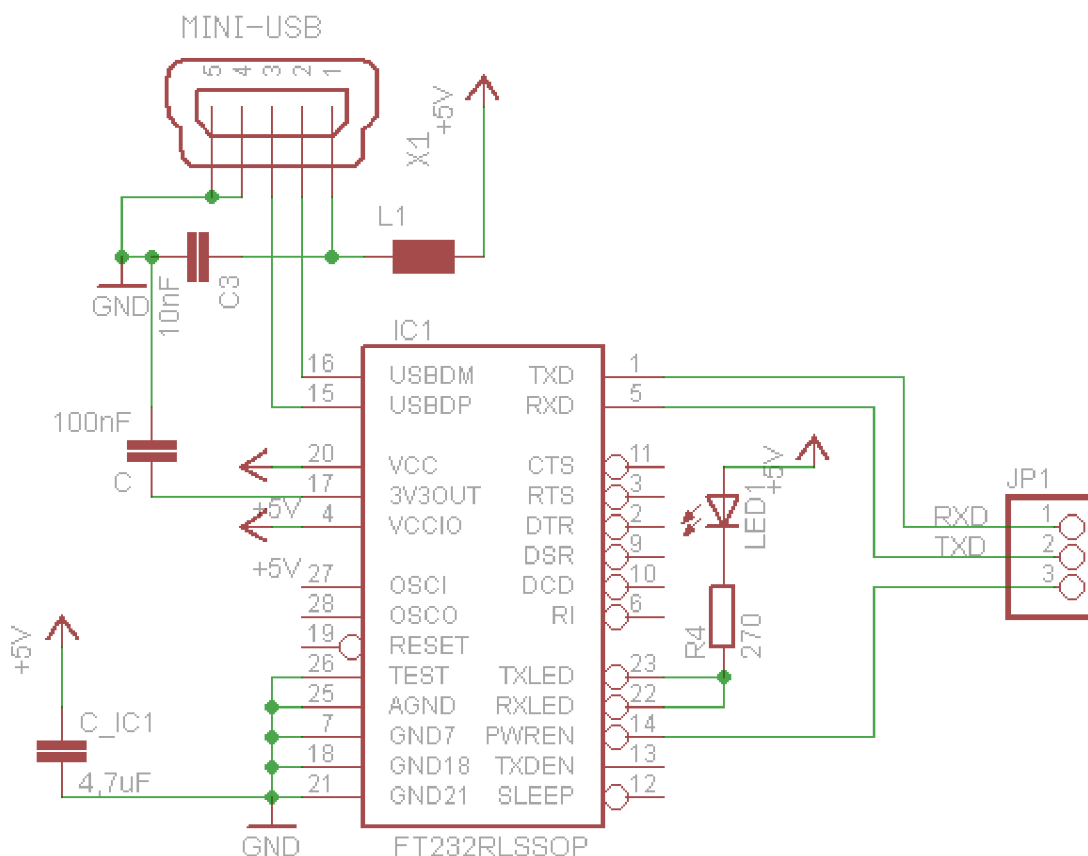
Obr. 5: Zapojení USB modulu
