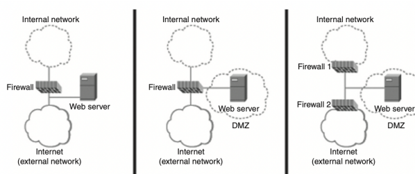
Obr. 4 Konfigurace DMZ
