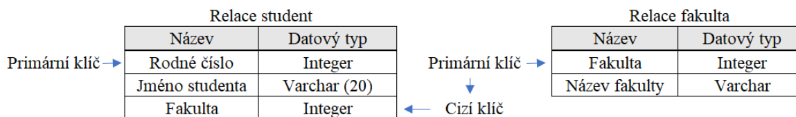
Obrázek č. 22: 3. normální forma po dekompozici (Zdroj: [1] s. 58)
