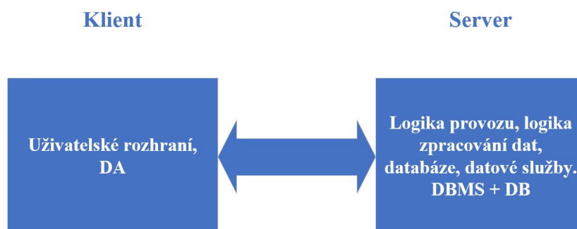
Obrázek č. 7: Architektura soustředěná na serveru (Zdroj: [6])
