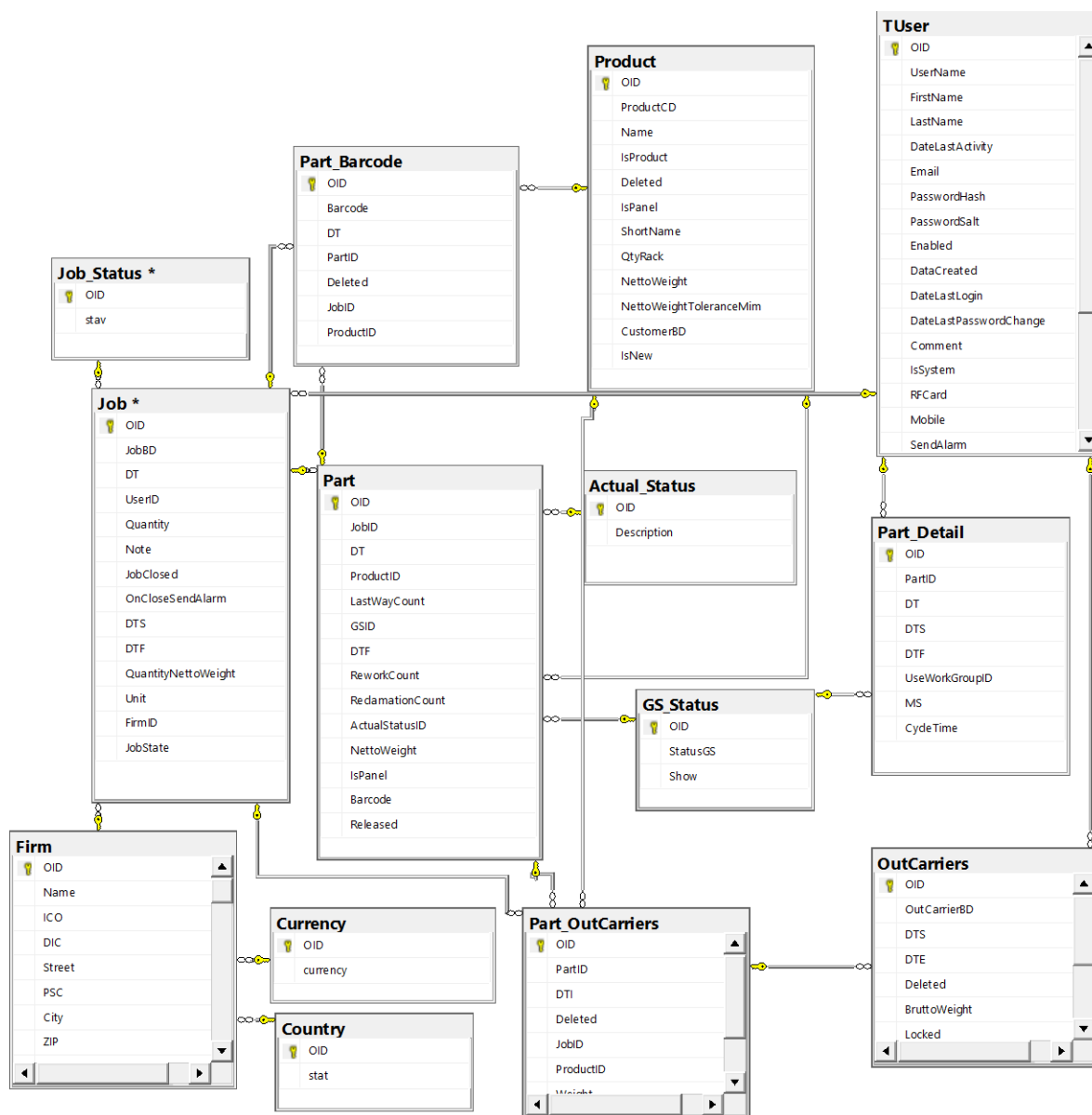
Obrázek č. 31: ER diagram databáze (Zdroj: vlastní zpracování)
