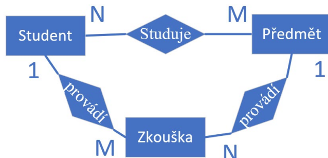
Obrázek č. 18: Vztah N:M po dekompozici (Zdroj: [1] s. 34)
