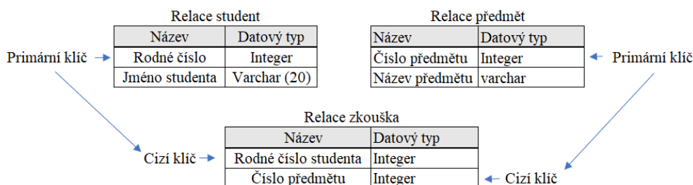
Obrázek č. 19: Vztah N:M po dekompozici v relacích (Zdroj: [1] s. 34)
