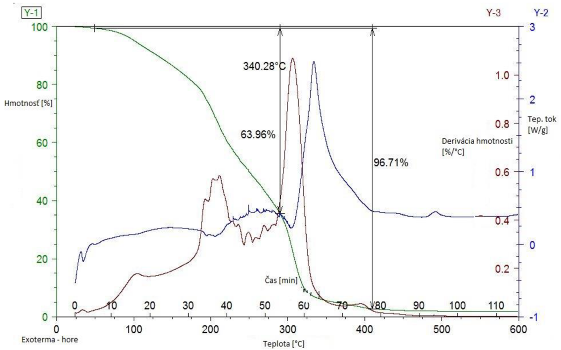
Obr. 32 – TGA a DTA analýza vzorky 10% EMIM vo vzduchu
