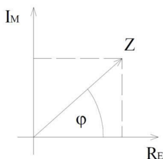
Obr. 3 – Reálna a imaginárna zložka impedancie
