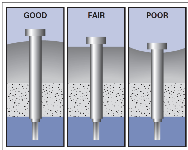
Obr. 4.2 Schéma vhodné úpravy terénu v okolí jímacího objektu [15]
