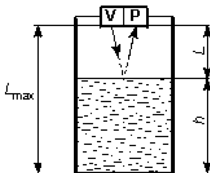
Obr. 4.15 Schéma ultrazvukového hladinoměru [32]
