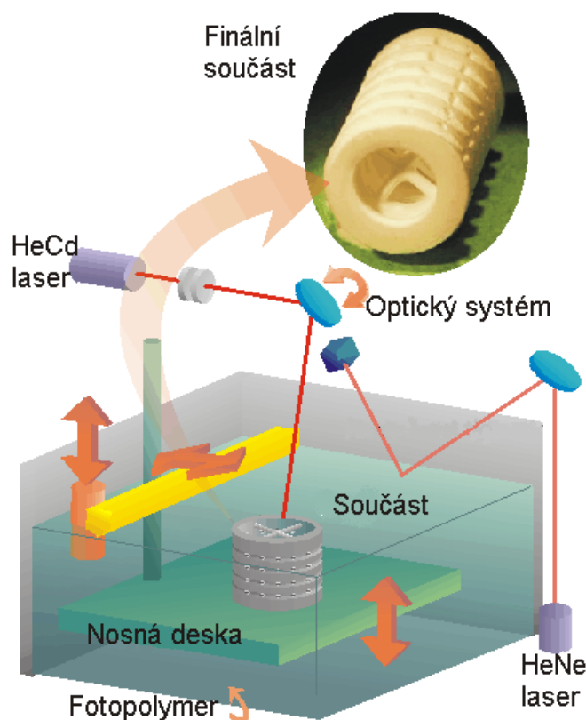
Obr. 1.3 Schéma stereolitografie (4)
