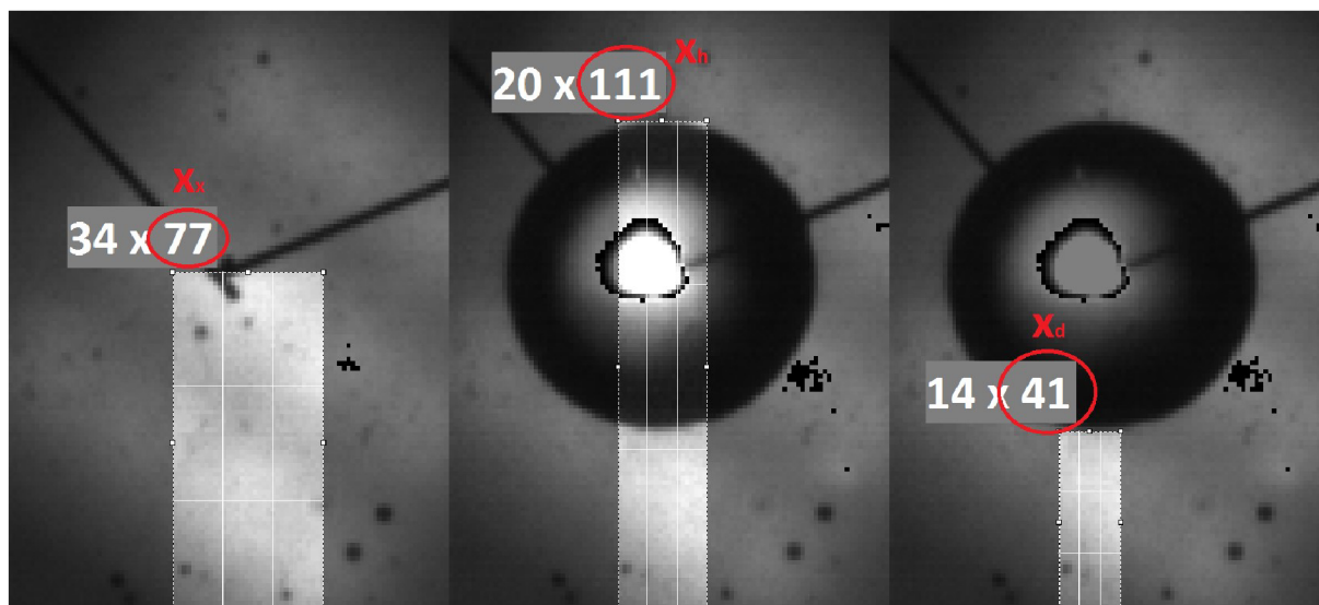
Obrázek 3.3 – měření vzdáleností styku elektrod, horního okraje a dolního okraje bubliny od spodního okraje snímku
