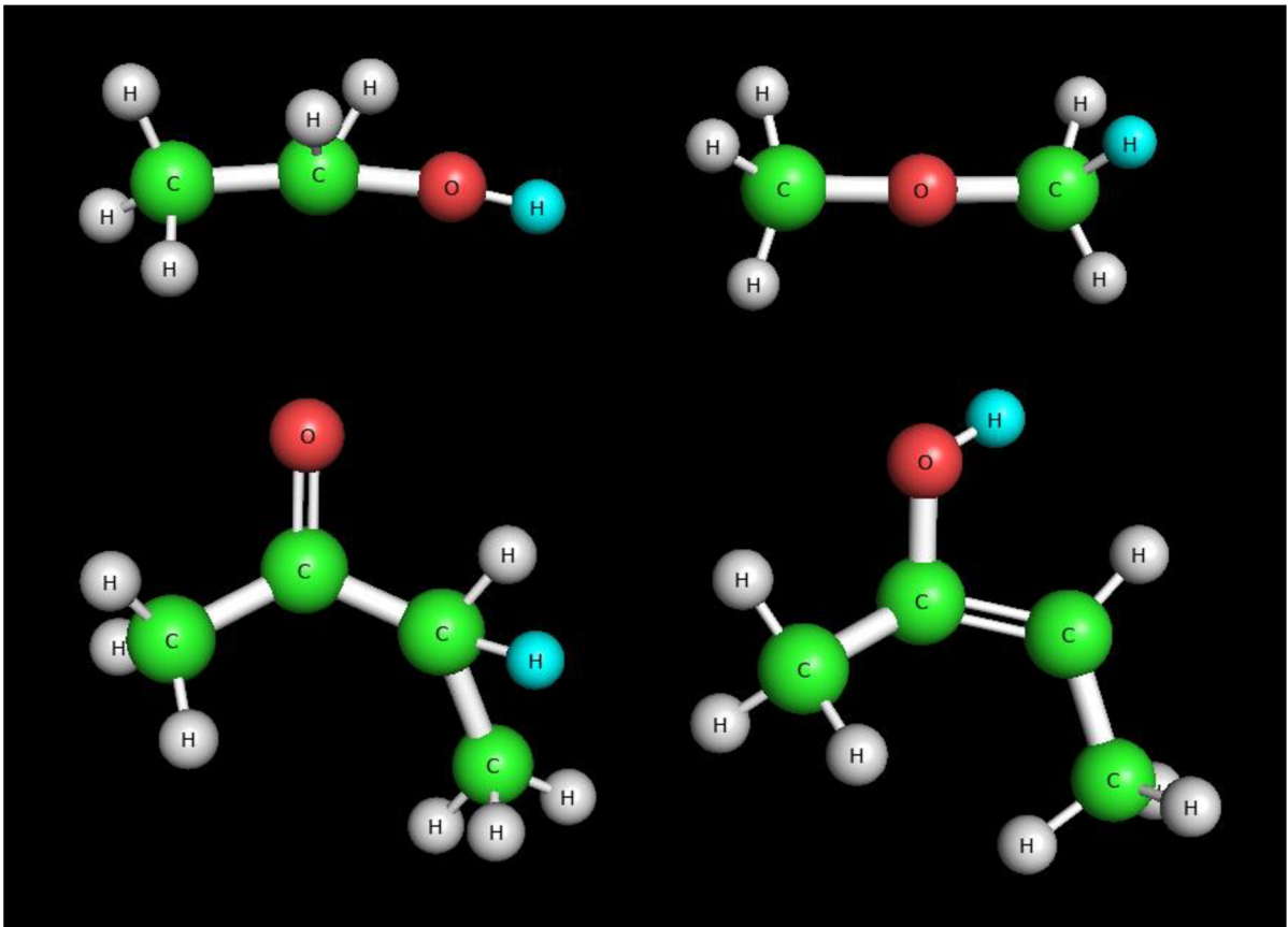
Zástupci skupinové izomerie: ethanol (vlevo nahoře) a dimethylether (vpravo nahoře); a keto-enol tautomerie : butan-2-on (vlevo dole) a but-2-en-2-ol (vpravo dole).
