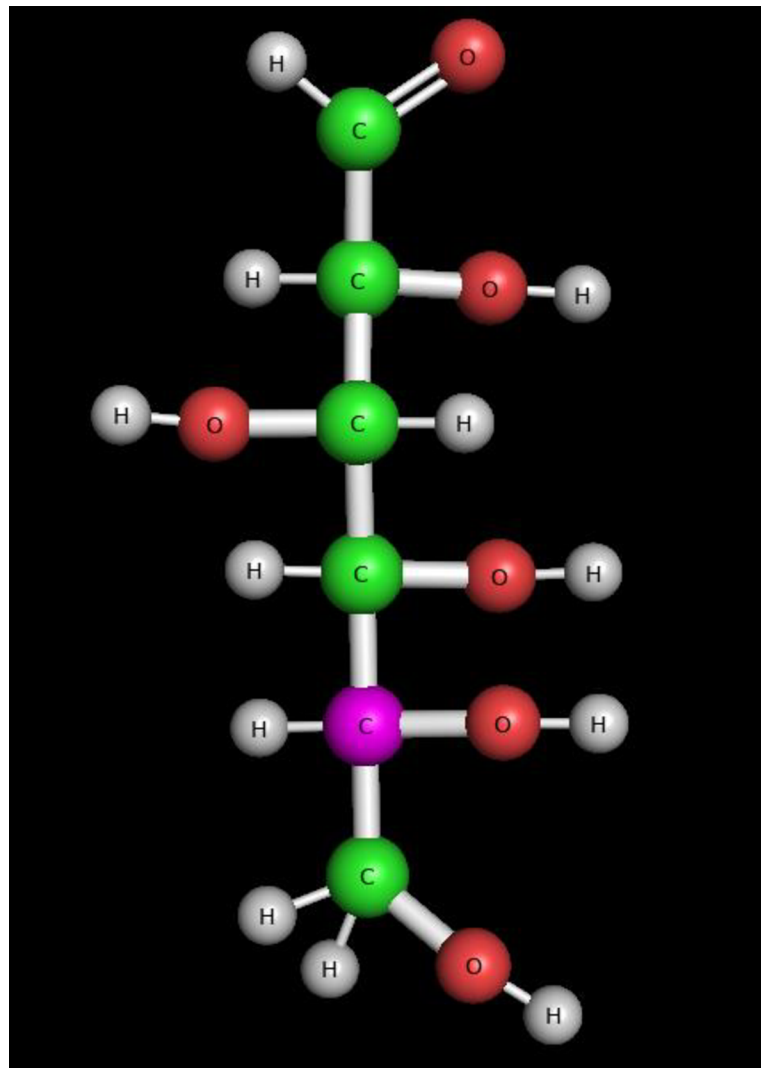
D-glukosa.
