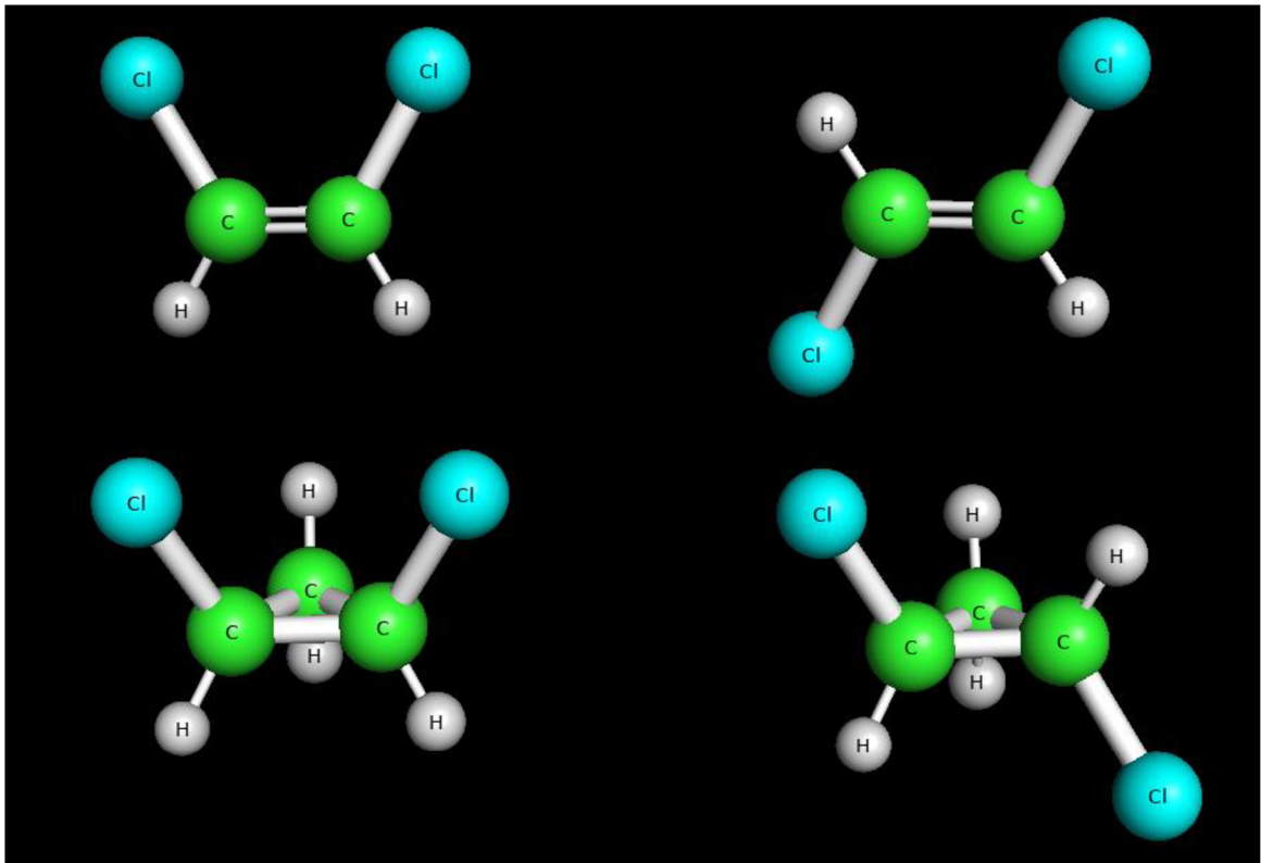
Zástupci geometrické izomerie : cis-1,2-dichlorethen (vlevo nahoře), trans-1,2-dichlorethen (vpravo nahoře), cis-1,2-dichlorcyklopropan (vlevo dole) a trans-1,2-dichlorcyklopropan (vpravo dole).
