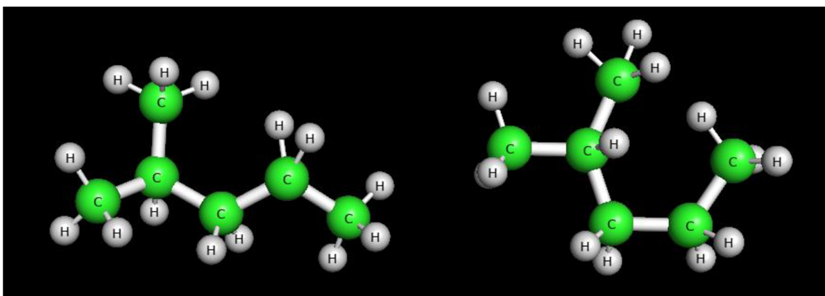
Konformační izomery 2-methylpentanu.
