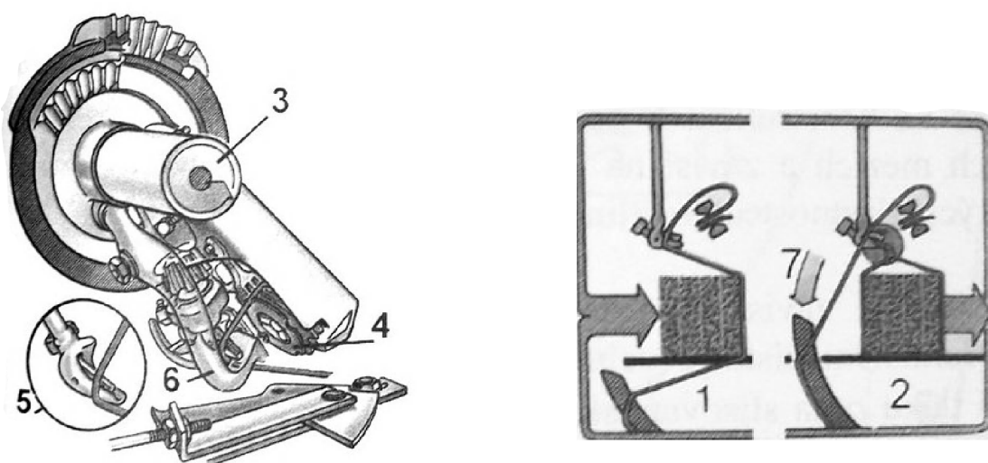
Obr. 3.22: Uzlovač typu Deering a činnost vázání: (1) tvoření balíku, (2) zavázání balíku, (3) hřdel uzlovačů, (4) svěrka, (5) roubík, (6) stahovač uzlů s nožkem, (7) jehla [2].
