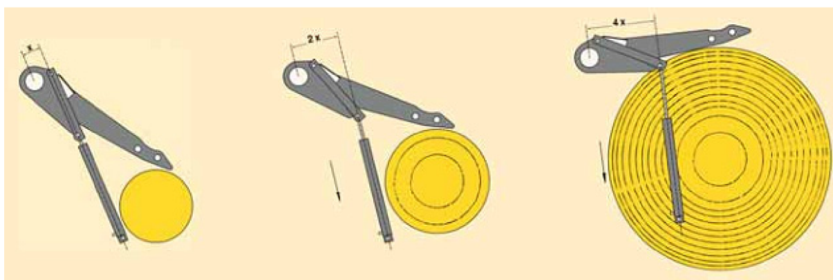
Obr. 4.3: Zvětšují se síla přítlaku pružin napínacího ramene při zvětšení velikosti průměru balíku [17].
