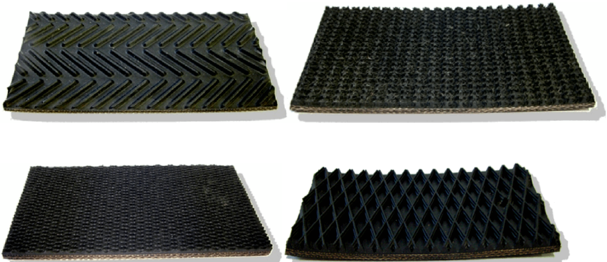
Obr. 4.7: Gumové pásy pro svinovací lisy fy Fomia – vlevo nahoře: střídavé vzorování určené pro suchý i vlhký materiál; vpravo nahoře: zdrsňené vzorování doporučené pro mokré materiály; vlevo dole: jemné vzorování pro suché materiály; vpravo dole: Kosočtverečný vzor pro univerzální použití [25].
