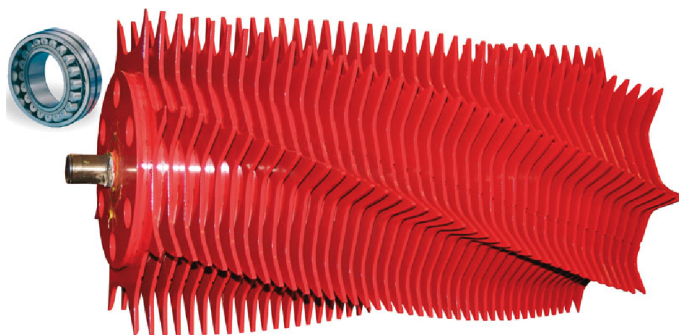
Obr. 3.11: Vkládací rotor fy Welger [20].
