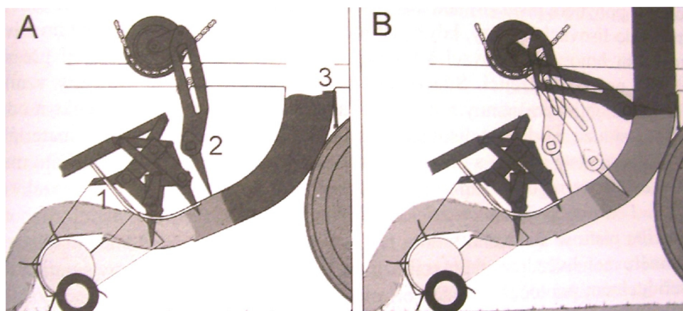
Obr. 3.16: Klikové pčhovací ústrojí [2].
