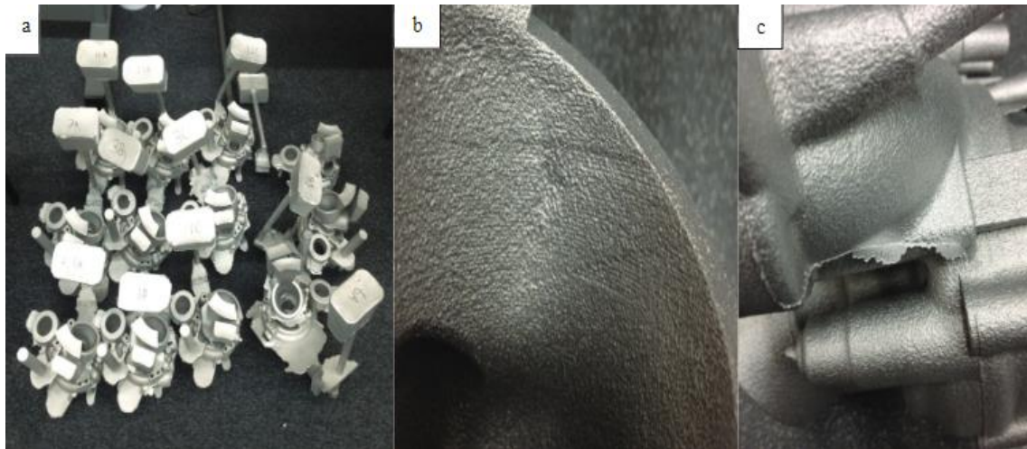
Obrázek 7: a) odlitky, b) a c) ukázka kvality povrchu odlitků [9]
