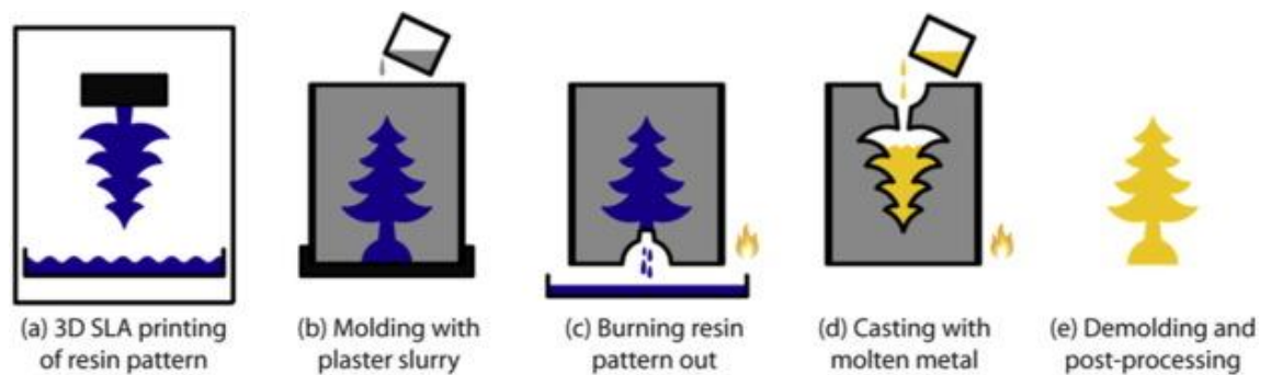
Obrázek 21: Postup výroby odlitku pomocí SLA [26]
