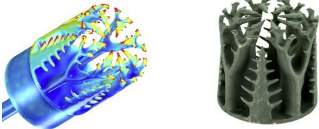
Obrázek 22: Výměník vyrobený aditivní technologií [26]
