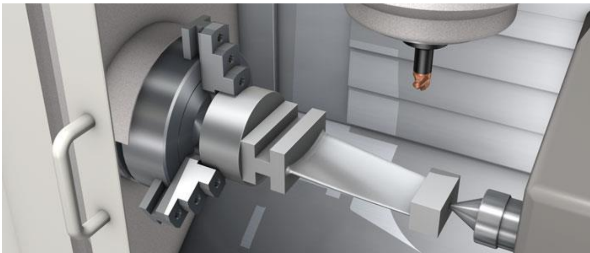
Obrázek 16: 5-ti osově obrábění turbínové lopatky [25]
