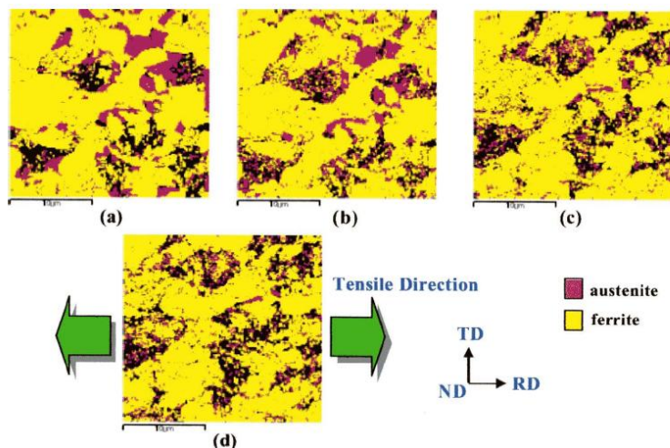
Obr.4.17 EBSD mapy in-situ deformované TRIP oceli [9].
