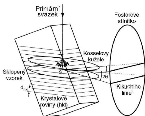
Obr.4.2 Vznik difrakčních pásů pomocí EBSD [1].
