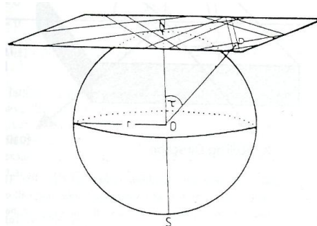
Obr.4.3 Kikuchiho obrazec jako gnómonická projekce difrakčních stop [1].
