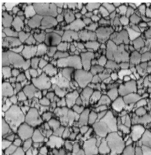
Obr.7.7 Mapa IQ nedeformovaného vzorku D5.
