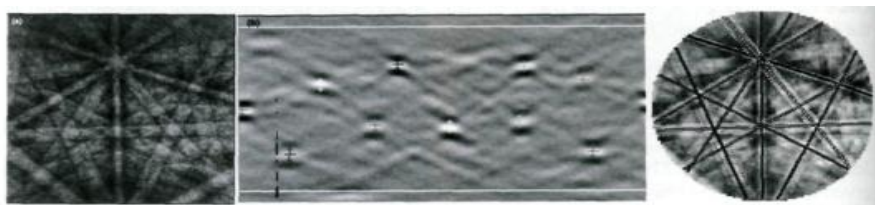
Obr.4.7 Obrázek Houghovy transformace a detekované pásy [1].
