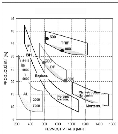
Obr. 2.1 Srovnání závislosti prodloužení na pevnosti pro jednotlivé typy ocelí [4].
