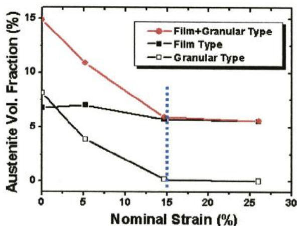
Obr.4.19 Vliv účinku deformace (in-situ) na podíl zbytkového austenitu [9].
