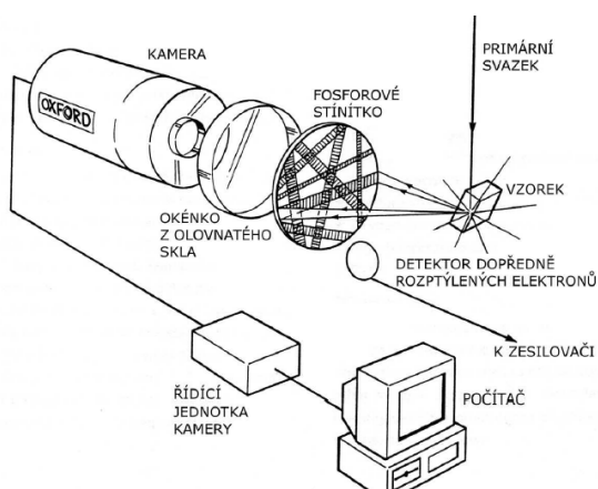
Obr.4.4 Schéma přístrojového řetězce pro snímání a zpracování difrakčních stop [2,3].
