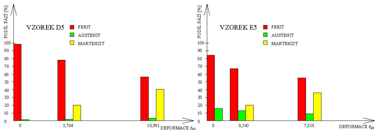
Obr. 7.33 Graf fázového složení jako funkce plastické deformace.
