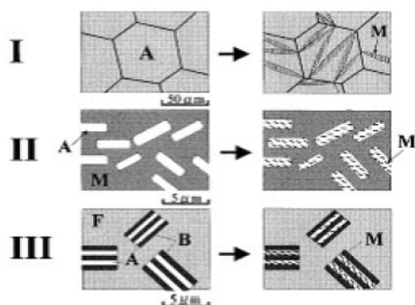
Obr.3.1 Schematické znázornění změny struktury u ocelí podporující TRIP efekt [4].
