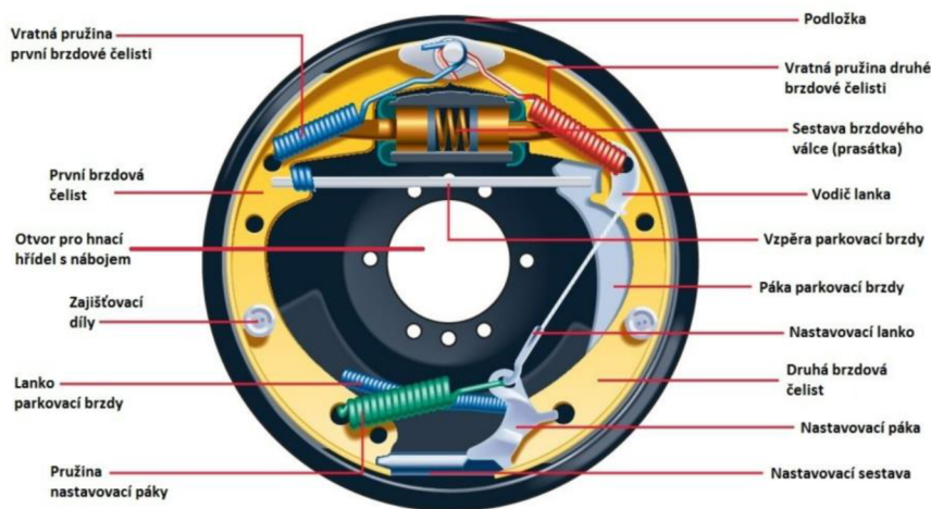
Obr.12 – Bubnová brzda [18]
