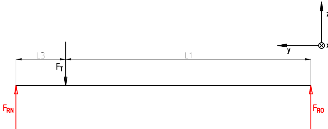
Obr.27 – Rozložení základních sil nápravy a tažného oka včetně těžiště (schematicky)
