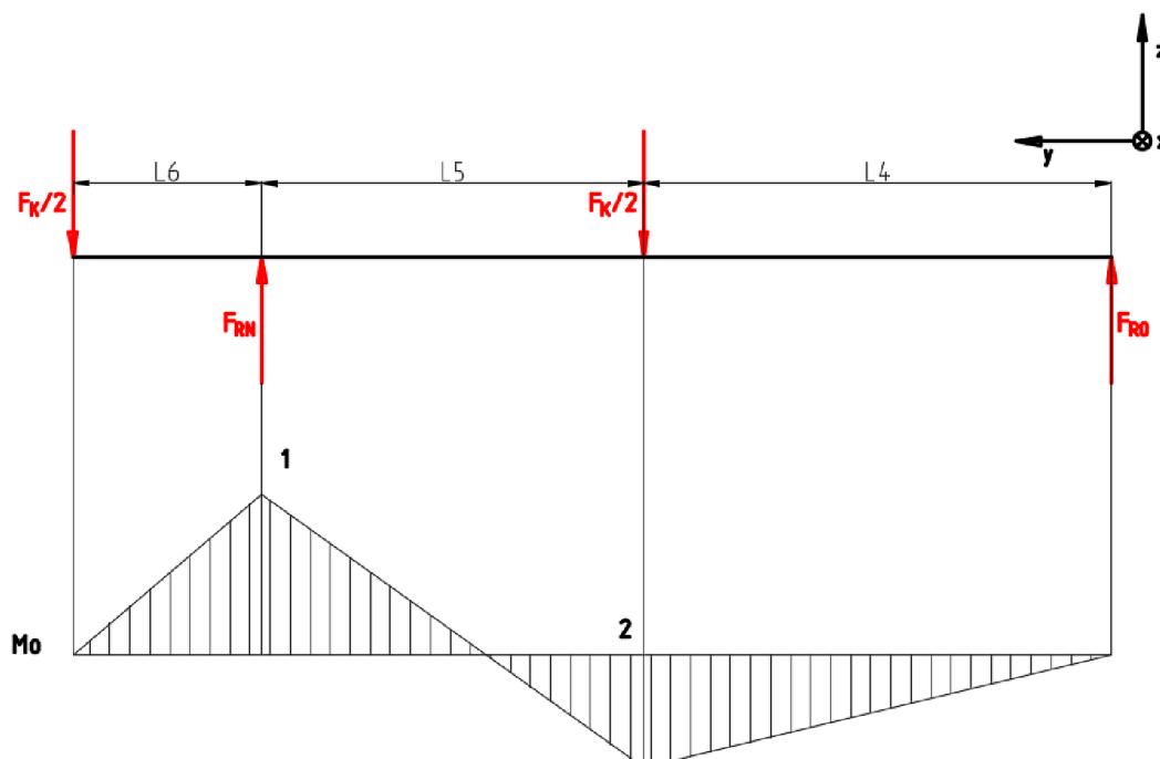
Obr.31 – Rozložení sil a průběh VVU v podélném směru (schematicky)
